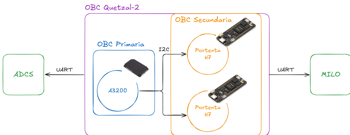
Figura 1: Diagrama de componentes de la OBC y sus protocolos de comunicación.
