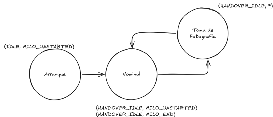
Figura 11: Estados de la OBC secundaria de estados finitos.
