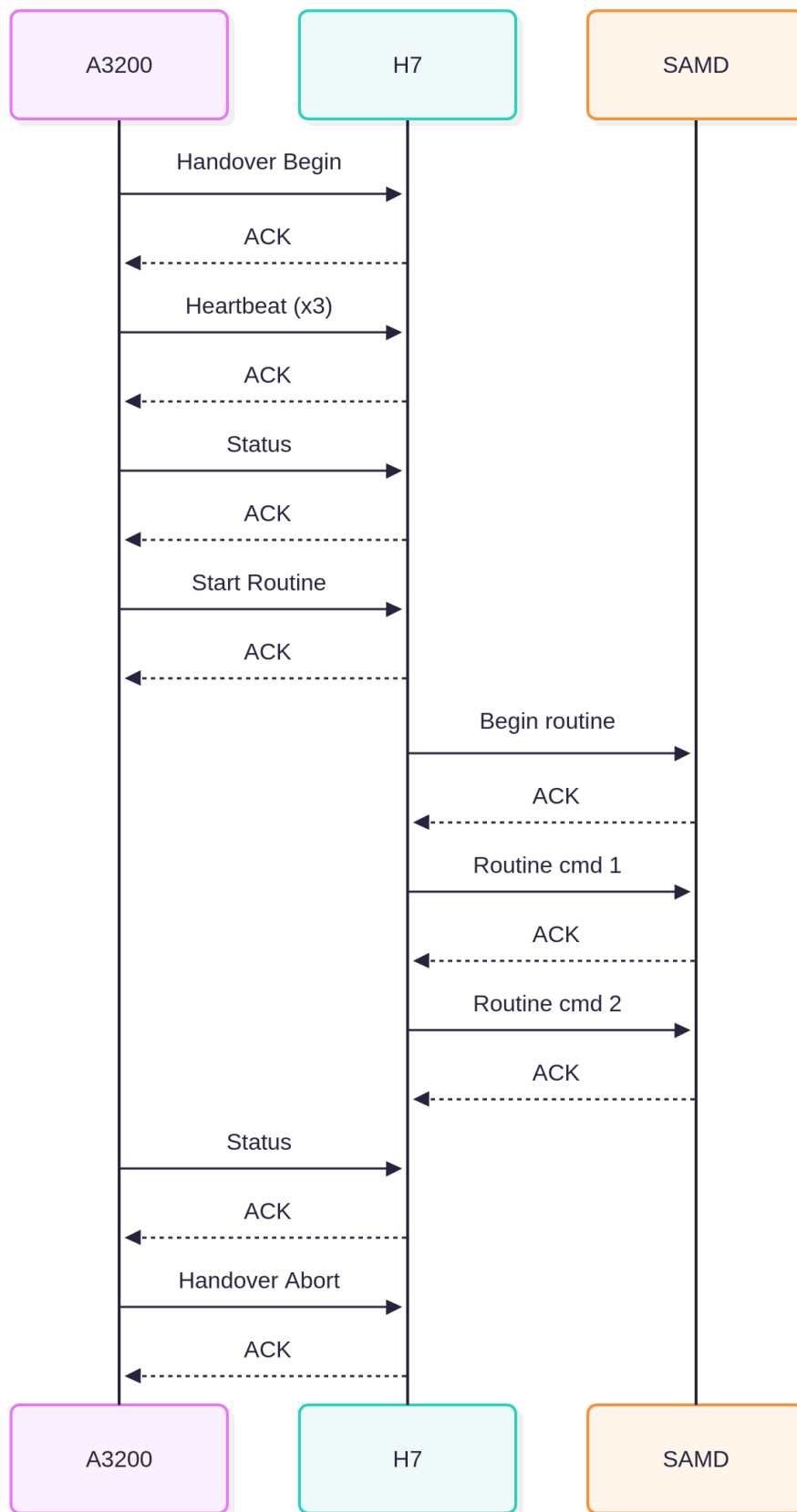
Figura 2: Diagrama de secuencia del protocolo de handover para un caso general.
