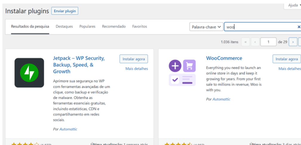
Figura 3 - instalação plugins
