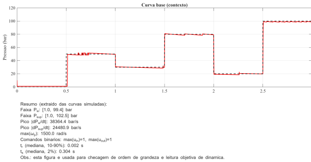
Figura 16. Resumo de ordens de grandeza (pressões, picos e tempos).
