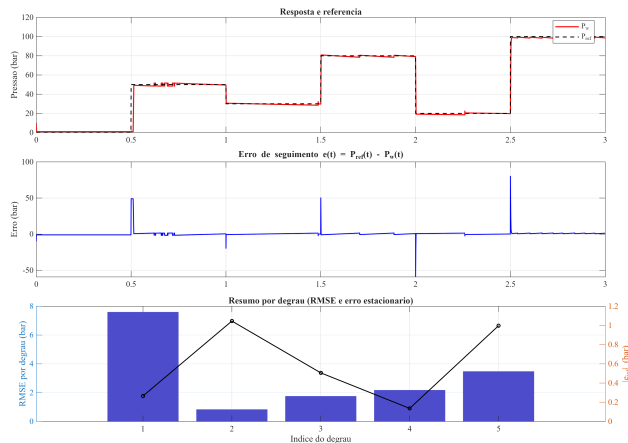
Figura 5. Seguimento por degraus: resposta e erro.
