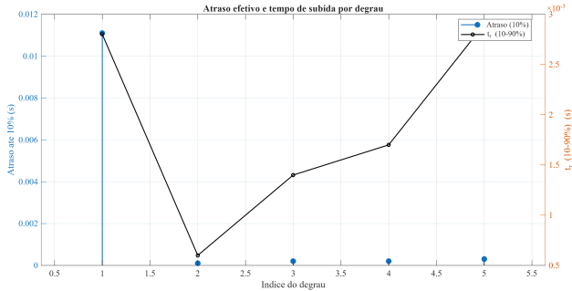
Figura 11. Atraso e tempo de subida por degrau.
