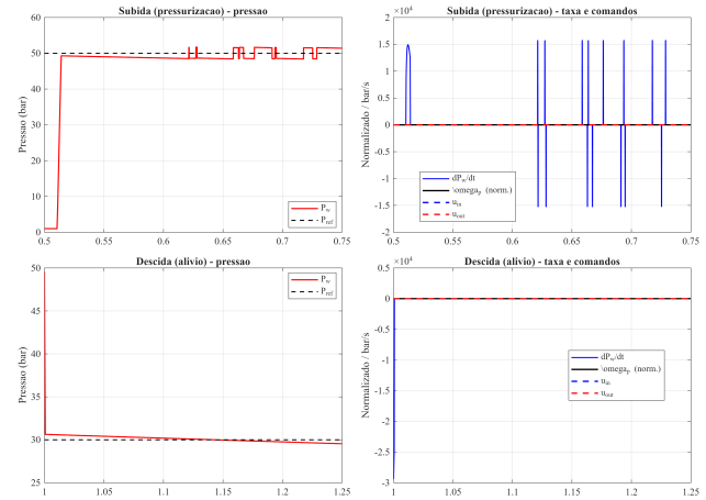
Figura 8. Pressurização vs. alívio: resposta e comandos.
