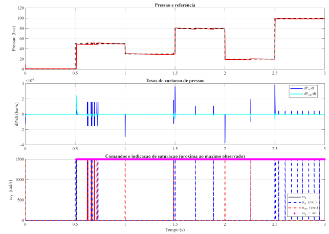
Figura 7. Taxas dP/dt e saturação do comando.
