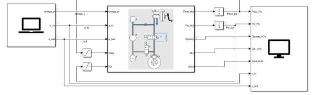
Figura 1. Circuito hidráulico: modelo concentrado em duas pressões.
