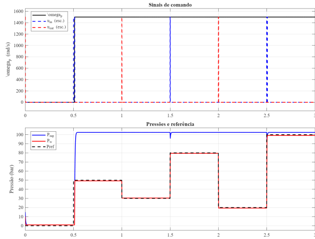
Figura 4. Malha fechada: pressão e comandos de atuação.
