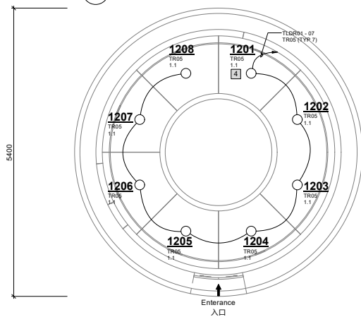
3 Space Elevator plan view (ceiling) - 太空电梯平面图(天花) 1:100
