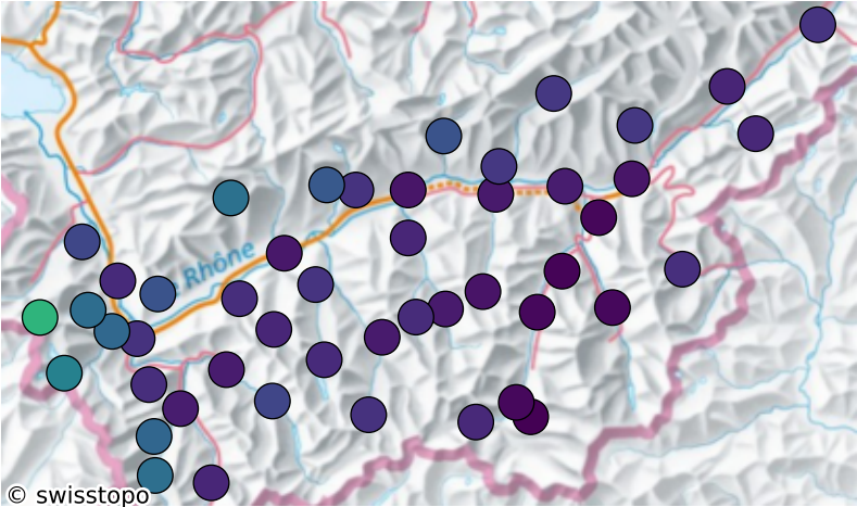
MLP
