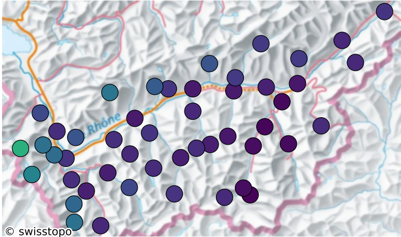
KAN
