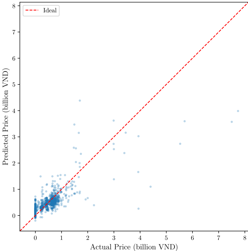
Lightgbm — Actual vs Predicted
