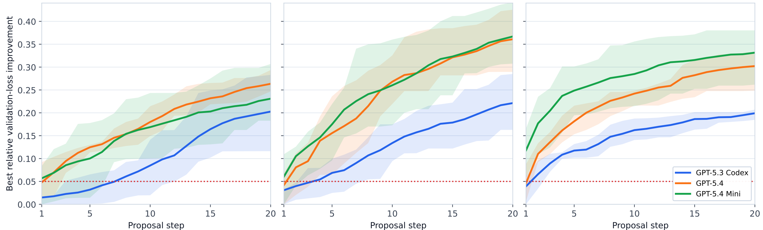
MLP
