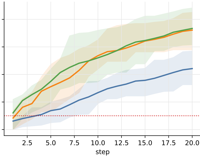
CNN
