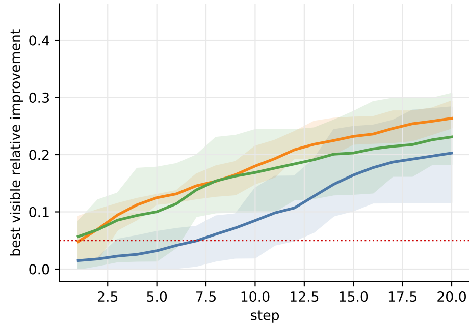
MLP
