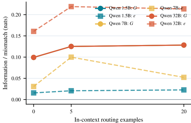
Posterior information and allocation mismatch
