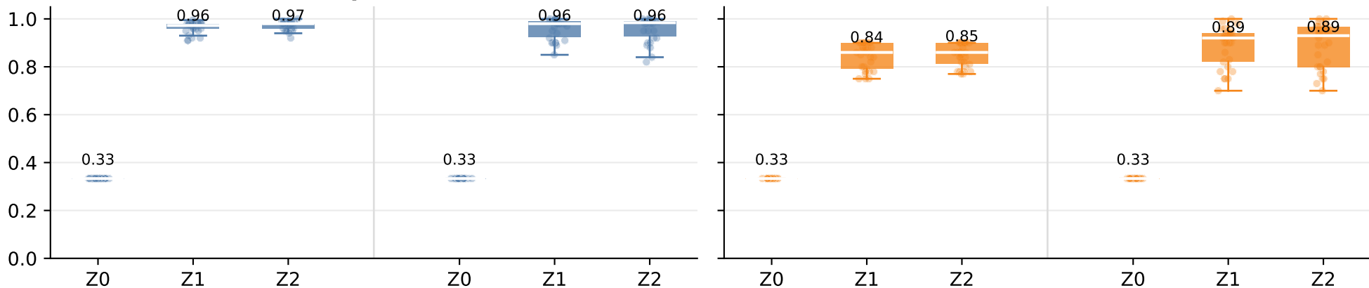
True-mode posterior mass
