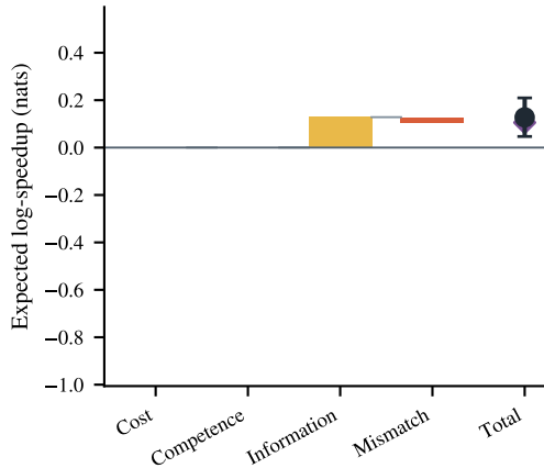
Qwen 1.5B
