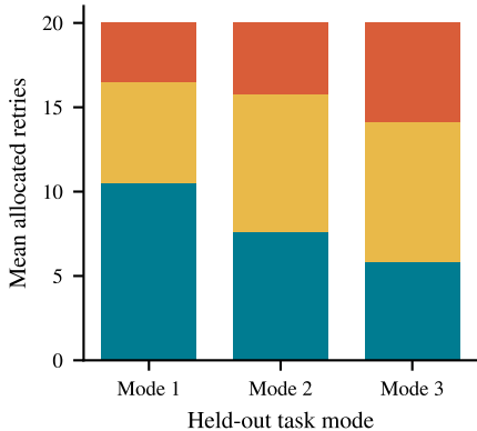
Qwen 1.5B
