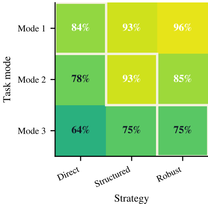
Qwen 1.5B
