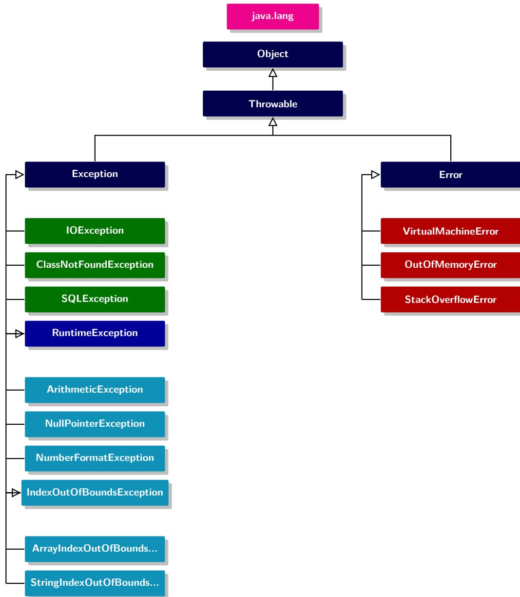
Figura 6.1: Gerarchia delle eccezioni in Java (Dettaglio UML)
