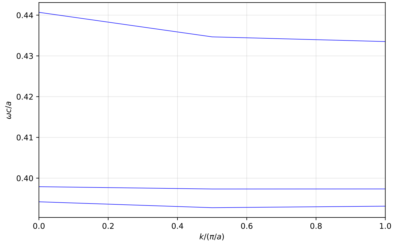
Estructura de bandas TE — barras plasmónicas
