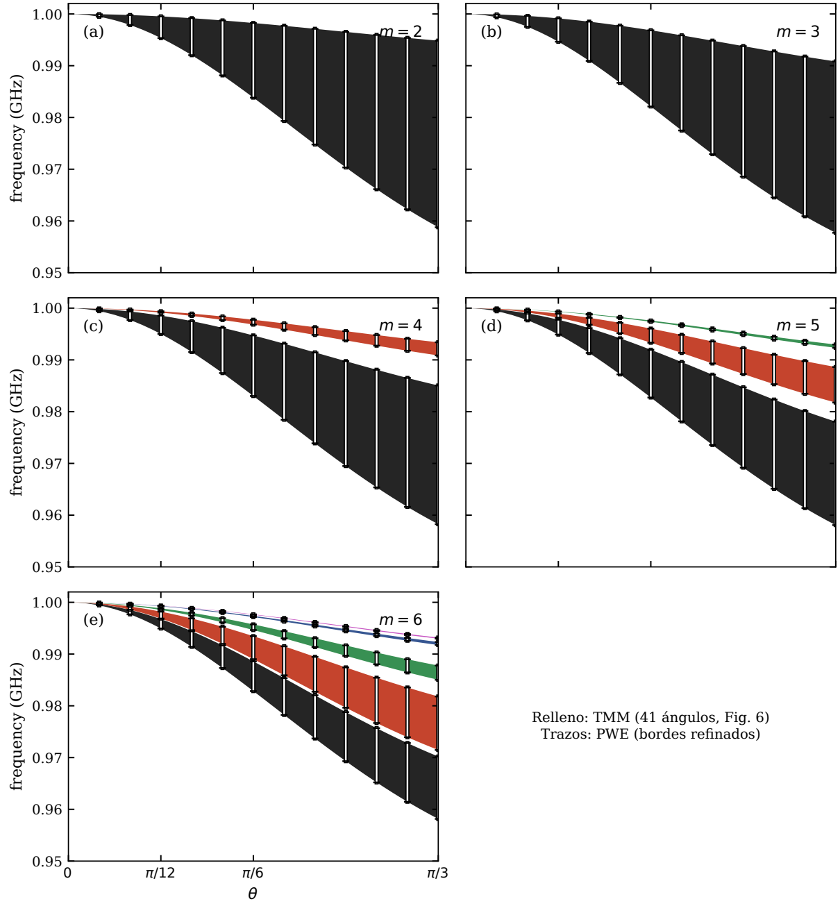
Figura 10: Fig. 6: subbandas frente al ángulo de incidencia. Relleno: la Fig. 6 de la TMM (41 ángulos); trazos blancos con topos: subbandas del PWE con bordes refinados (12 ángulos, \theta = 5^\circ \dots 60^\circ ). Cada color es una subbanda.
