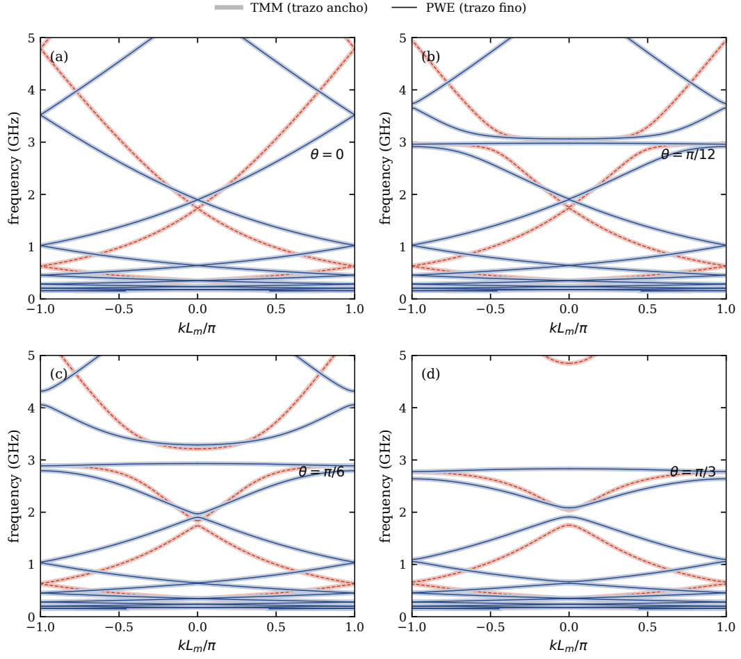
Figura 1: Fig. 1: relación de dispersión TMM (trazo ancho) y PWE (trazo fino) para m = 3 (rojo, discontinuo) y m = 4 (azul) en cuatro ángulos.
