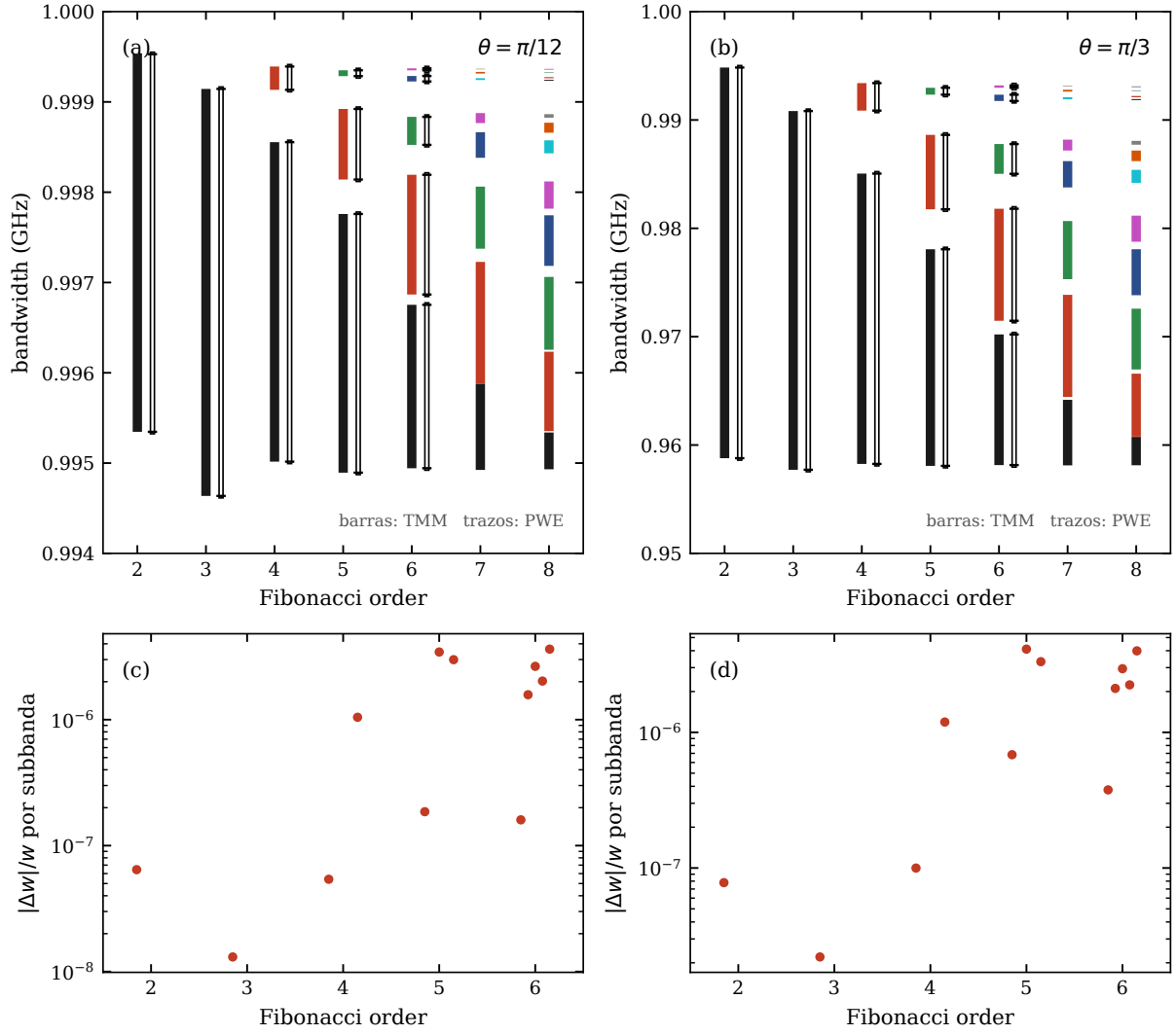
Figura 9: Fig. 5. Arriba: intervalos permitidos debajo de \nu_m para cada orden m ; las barras de colores son las de la Fig. 5 de la TMM y el trazo blanco con topes a su derecha es la subbanda del PWE. Los órdenes m = 7, 8 solo se calculan con la TMM. Abajo: error relativo del ancho de cada subbanda del PWE respecto a la TMM.
