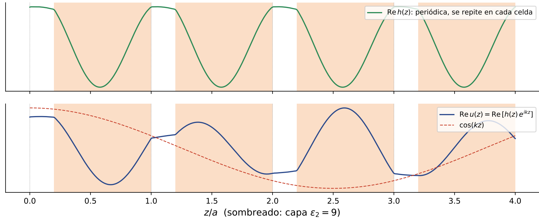
Modo de Bloch, banda 2, ka = 0.4\pi , \omega a/2\pi c = 0.293
