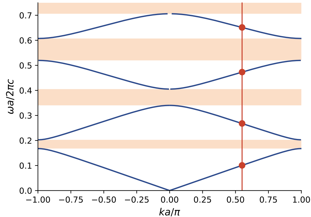
\omega(k) : fijo k , busco los \omega (libro)
