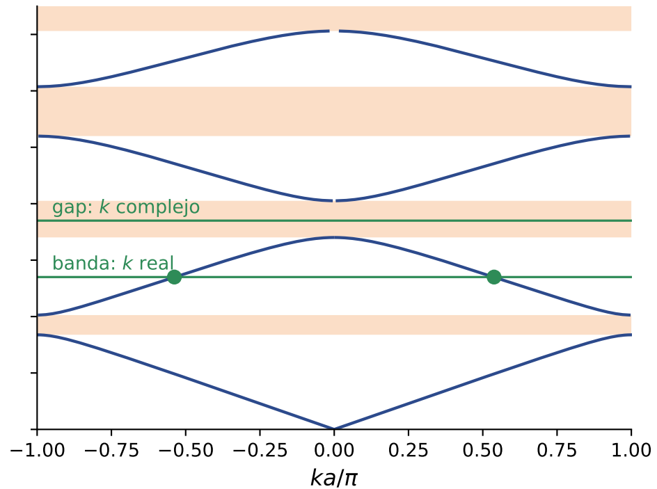
k(\omega) : fijo \omega , busco k (proyecto)
