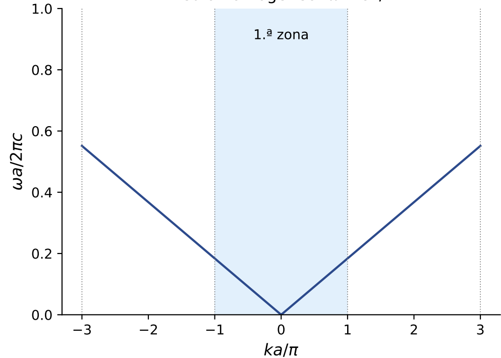
Medio homogéneo: \omega = ck/\bar{n}
