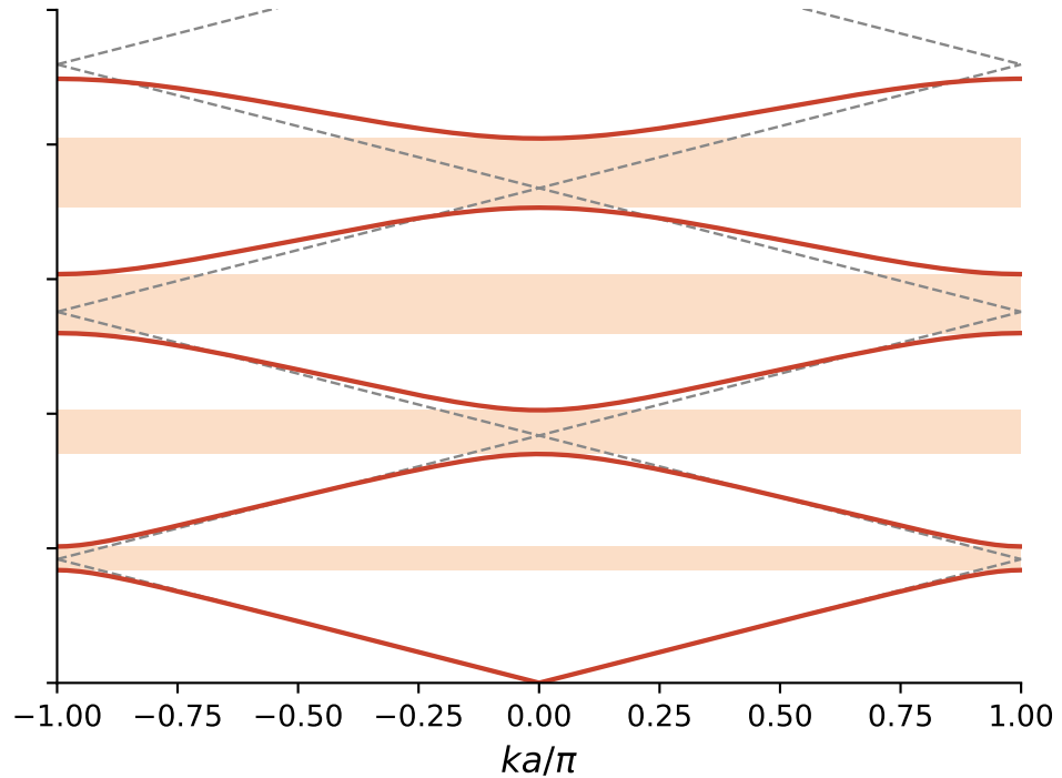
Plegado (gris) y cristal real (rojo): gaps
