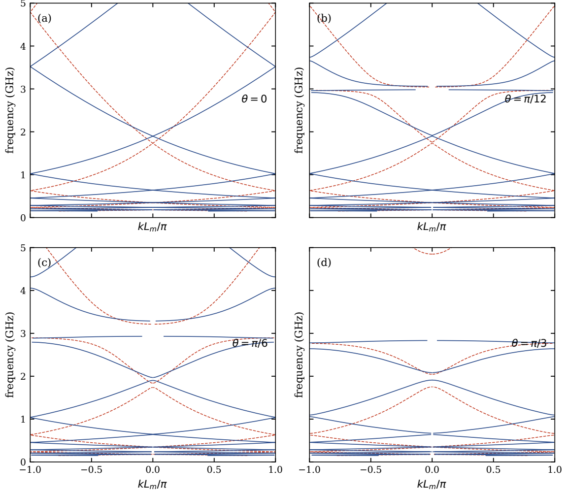
Figura 1: Reproducción de la Fig. 1. Dispersión TE para S_3 (discontinuo) y S_4 (continuo). Script: scripts/reproduce_figure_01.py .
