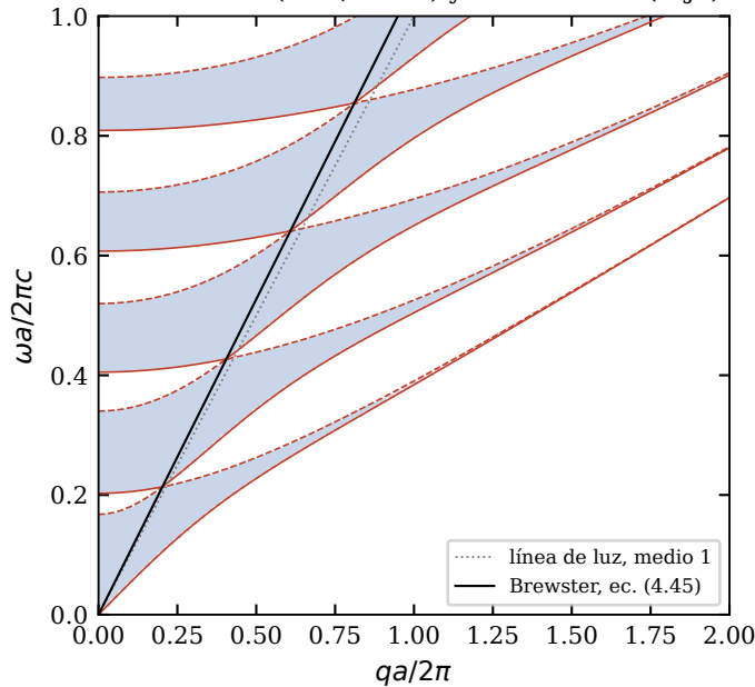
TM: bandas (azul, TMM) y bordes PWE (rojo)
