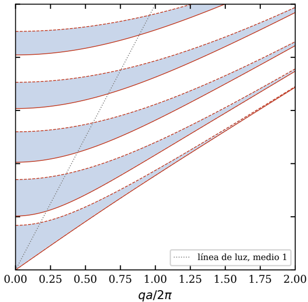
TE: bandas (azul, TMM) y bordes PWE (rojo)
