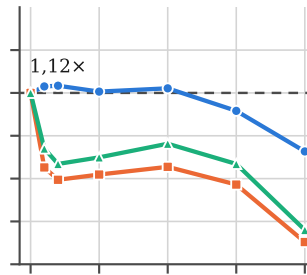
soc-LiveJournal1
