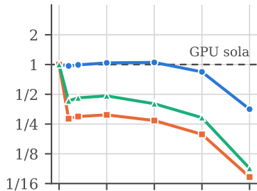
cit-Patents
