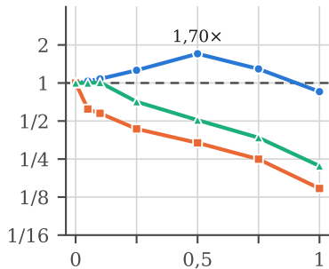
cit-Patents
