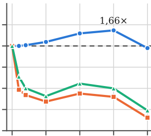
wiki-topcats
