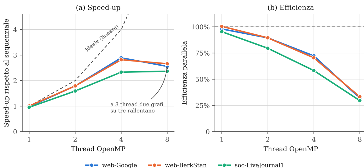
Figura 1: Scalabilità della versione OpenMP. Il riferimento per lo speed-up è la build sequenziale vera, compilata senza -fopenmp . La linea tratteggiata in (a) indica lo speed-up lineare ideale; in (b) l'efficienza del 100 %. Su web-Google e web-BerkStan il passaggio da 4 a 8 thread peggiora il tempo di esecuzione. Figura generata da tools/plot_results.py a partire da results/bench.csv .
