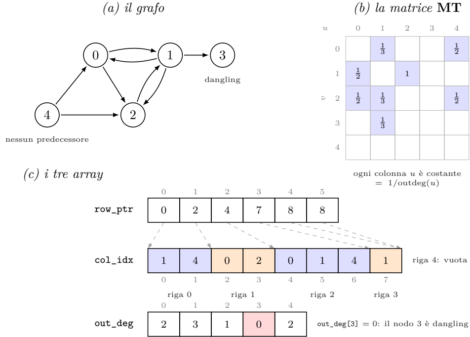
Figura 1: Costruzione del CSR trasposto su un grafo con N = 5 nodi e M = 8 archi. In (b) la riga v della matrice \mathbf{MT} raccoglie i predecessori di v , e ogni colonna u ha il valore costante 1/\text{outdeg}(u) . In (c) col_idx concatena le righe di (b), row_ptr[v] indica dove ciascuna comincia (le frecce tratteggiate) e out_deg conserva i denominatori. Le due condizioni limite sono distinte e vivono su array distinti: la riga 4 è vuota perché nessuno punta al nodo 4, mentre out_deg[3] è nullo perché il nodo 3 non ha archi uscenti.
