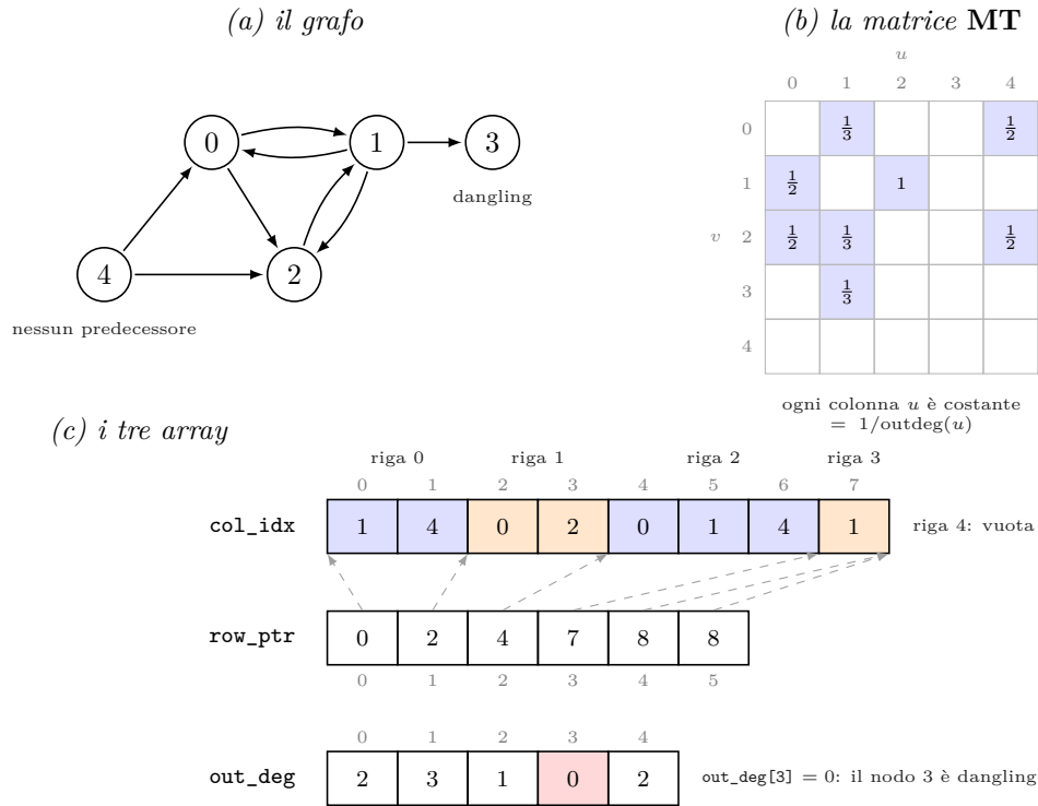
Figura 1: Costruzione del CSR trasposto su un grafo con N = 5 nodi e M = 8 archi. In (b) la riga v della matrice \mathbf{MT} raccoglie i predecessori di v , e ogni colonna u ha il valore costante 1/\text{outdeg}(u) . In (c) col_idx concatena le righe di (b), row_ptr[v] indica dove ciascuna comincia (le frecce tratteggiate) e out_deg conserva i denominatori. Le due condizioni limite sono distinte e vivono su array distinti: la riga 4 è vuota perché nessuno punta al nodo 4, mentre out_deg[3] è nullo perché il nodo 3 non ha archi uscenti.
