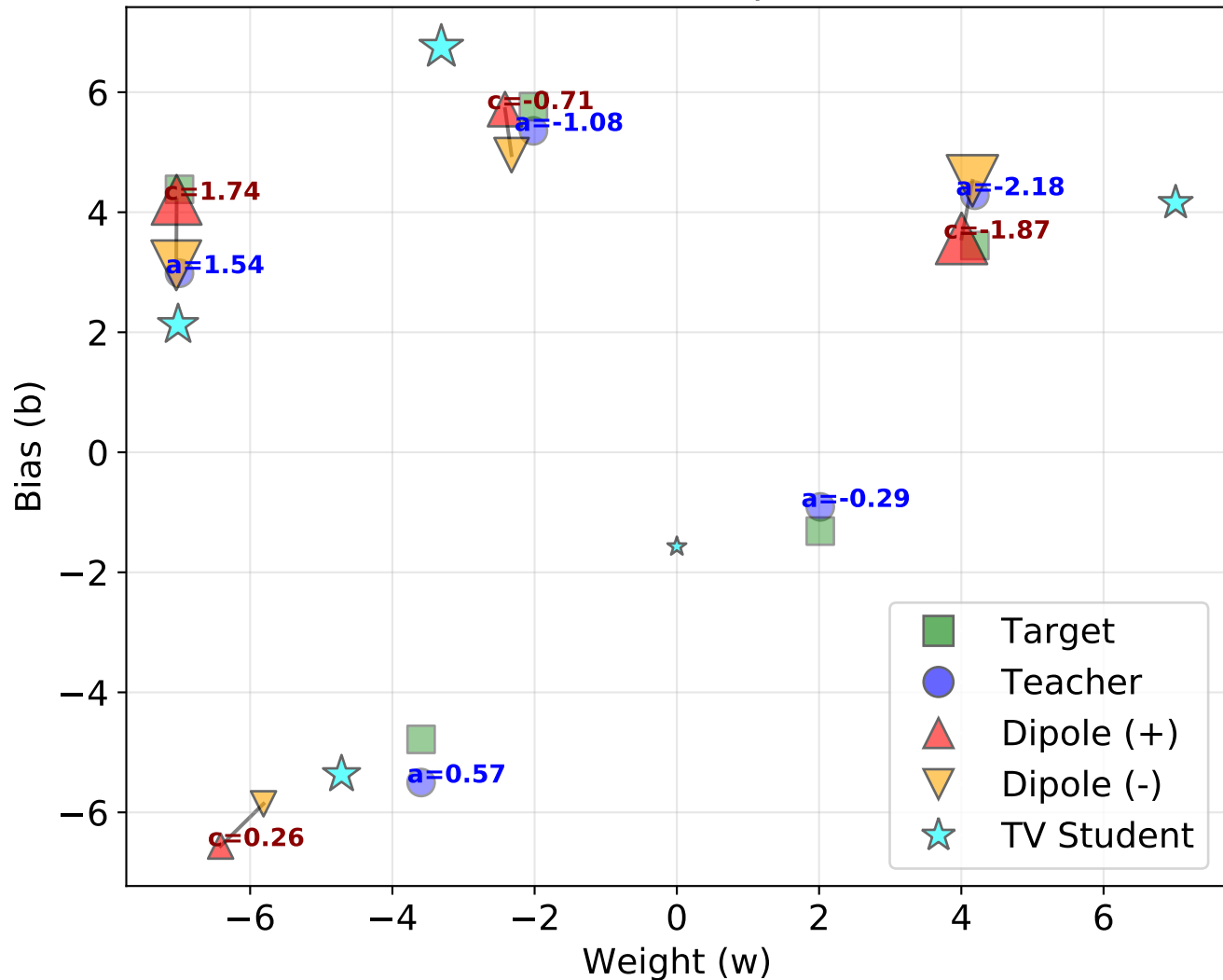
Parameter Space
