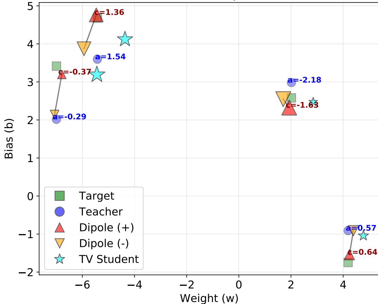
Parameter Space
