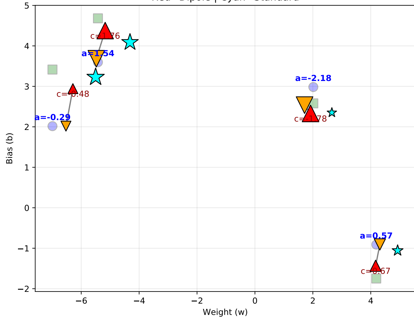
Parameter Space Red=Dipole | Cyan=Standard
