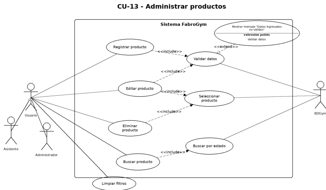
Figura 33: Diagrama UML monocromatico detallado de CU-13: Administrar productos.
