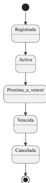
Figura 65: Estados de la membresia.
