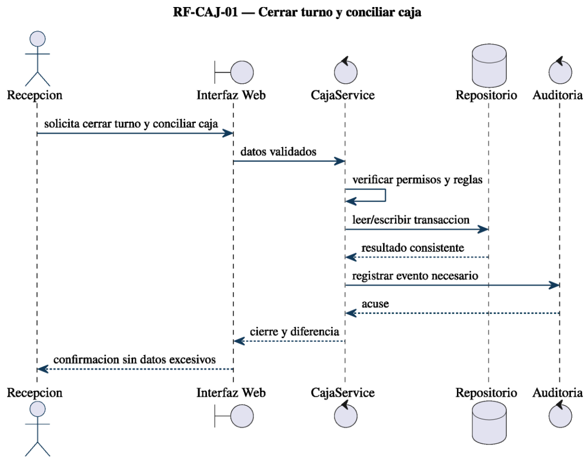
Figura 56: Diagrama de secuencia de RF-CAJ-01: cerrar turno y conciliar caja.
