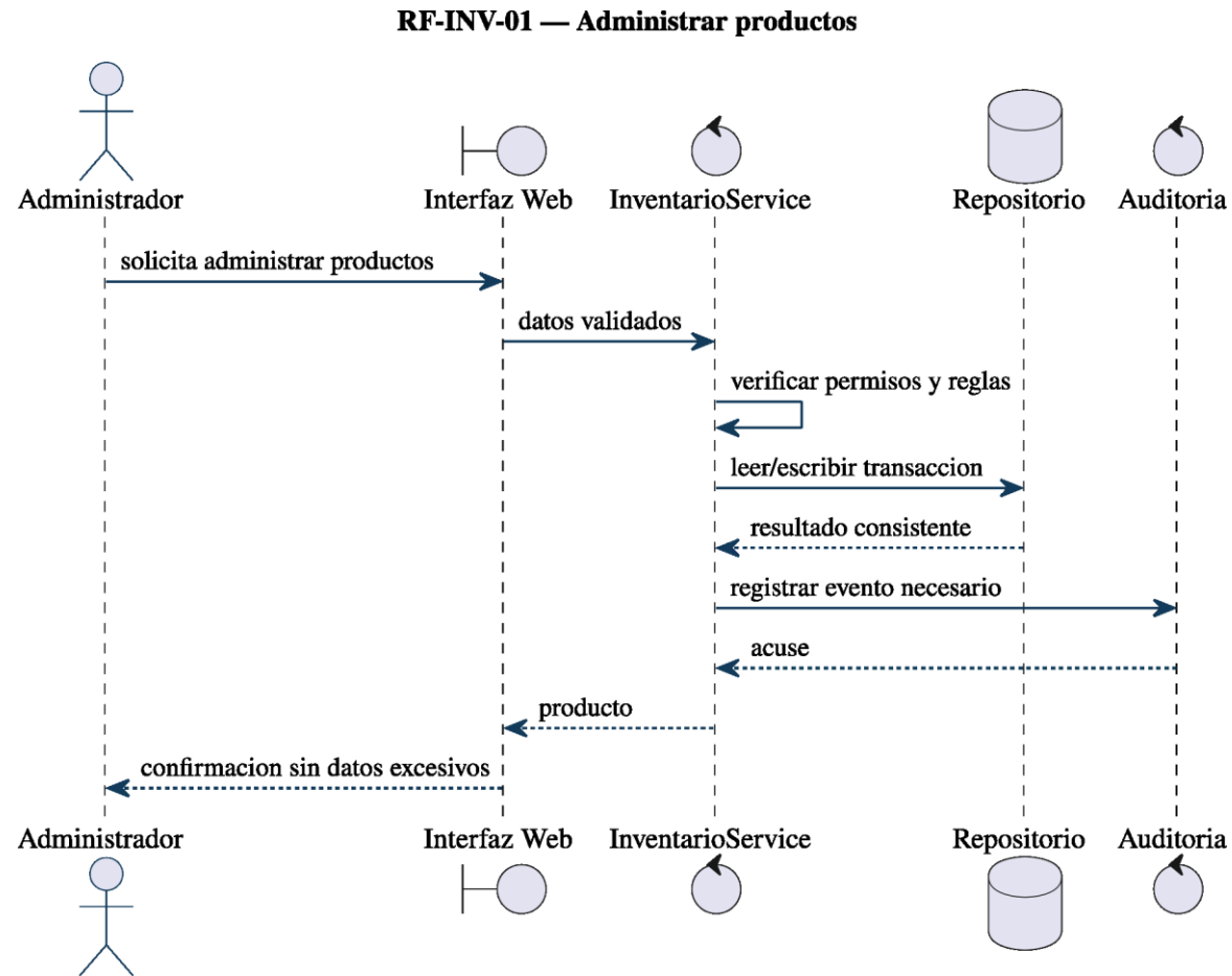
Figura 53: Diagrama de secuencia de RF-INV-01: administrar productos.
