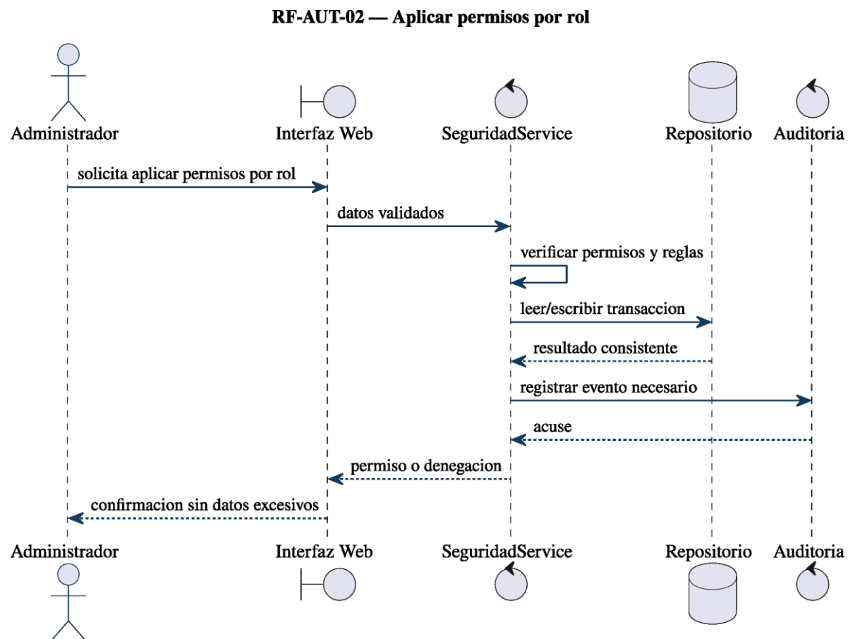
Figura 42: Diagrama de secuencia de RF-AUT-02: aplicar permisos por rol.
