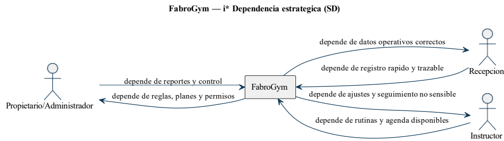
Figura 3: Dependencias estrategicas (SD).
