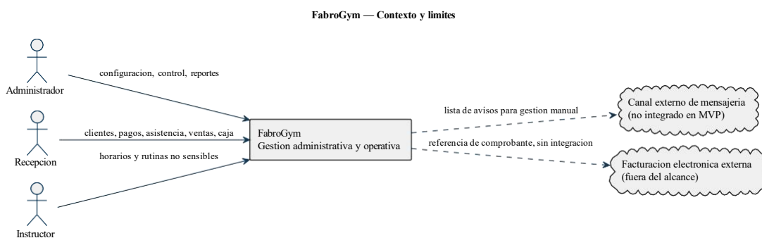
Figura 1: Contexto y límites del sistema.
