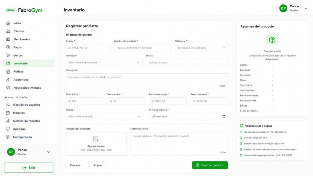
Figura 15: MU-28: Registro de producto y stock minimo. Rol: Dueño/Administrador. RF: RF-INV-01.
