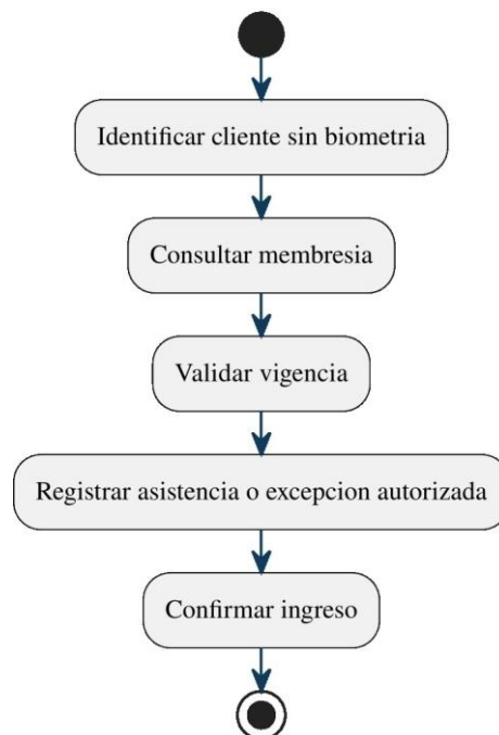
Figura 61: Actividad de ingreso y registro de asistencia.
