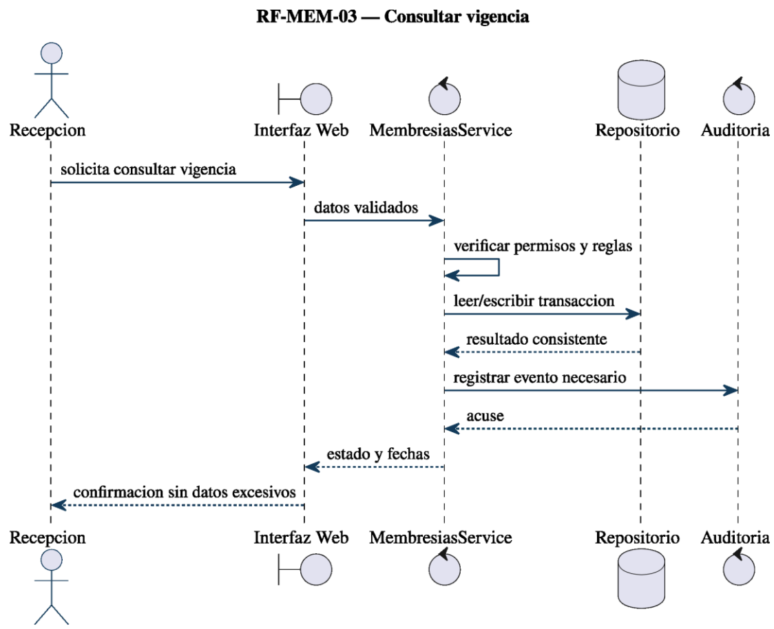
Figura 48: Diagrama de secuencia de RF-MEM-03: consultar vigencia.
