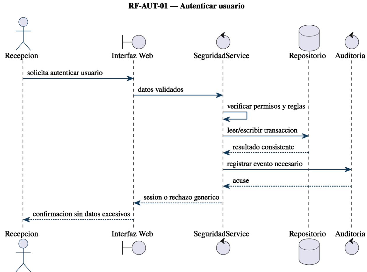
Figura 41: Diagrama de secuencia de RF-AUT-01: autenticar usuario.
