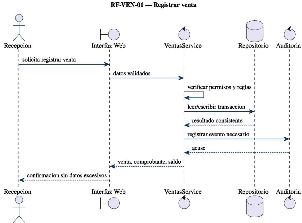
Figura 55: Diagrama de secuencia de RF-VEN-01: registrar venta.
