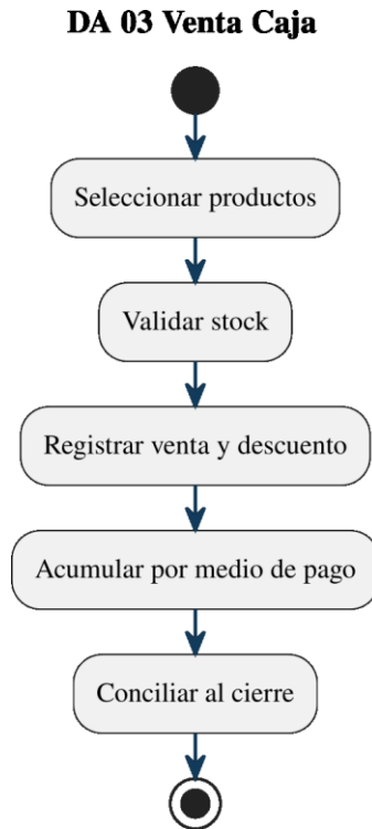
Figura 62: Actividad de venta y caja.
