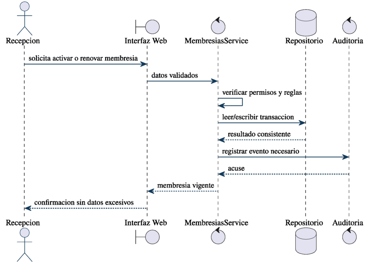
Figura 47: Diagrama de secuencia de RF-MEM-02: activar o renovar membresia.
