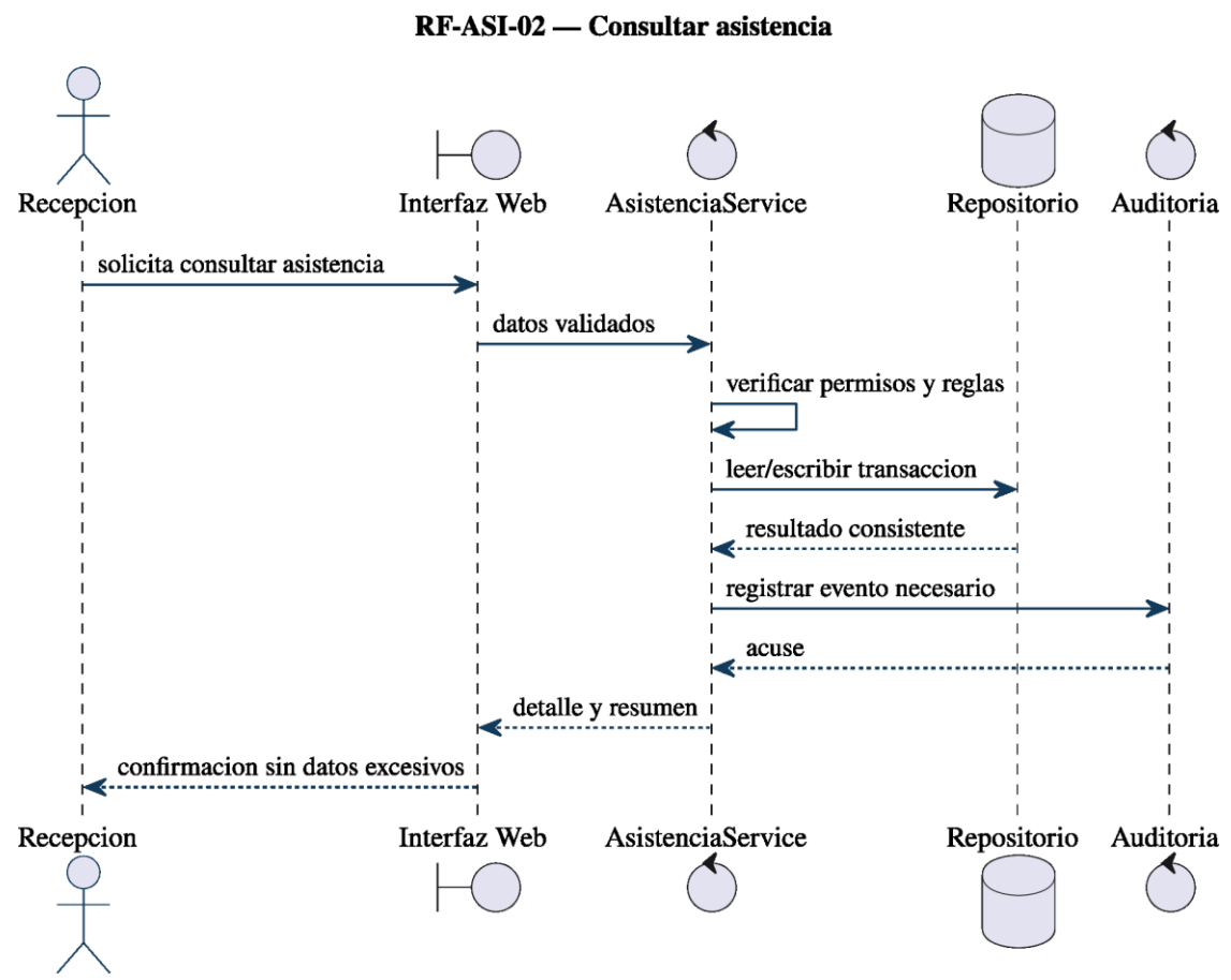
Figura 52: Diagrama de secuencia de RF-ASI-02: consultar asistencia.
