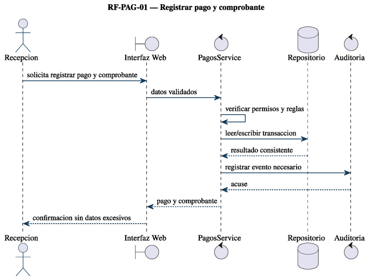
Figura 50: Diagrama de secuencia de RF-PAG-01: registrar pago y comprobante.
