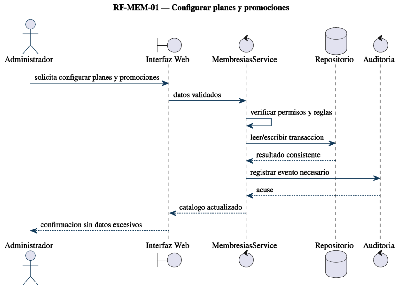
Figura 46: Diagrama de secuencia de RF-MEM-01: configurar planes y promociones.
