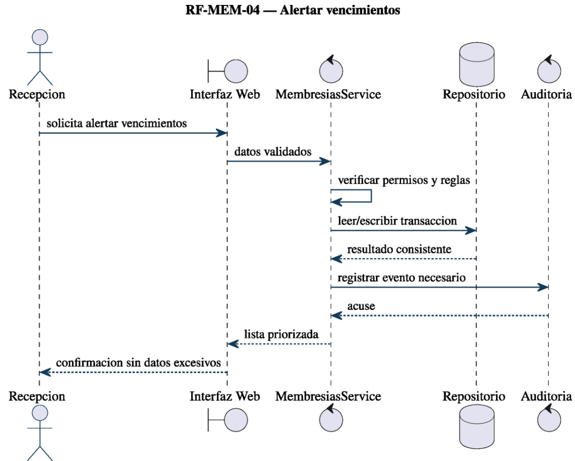
Figura 49: Diagrama de secuencia de RF-MEM-04: alertar vencimientos.
