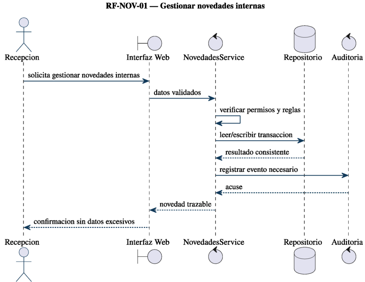
Figura 57: Diagrama de secuencia de RF-NOV-01: gestionar novedades internas.
