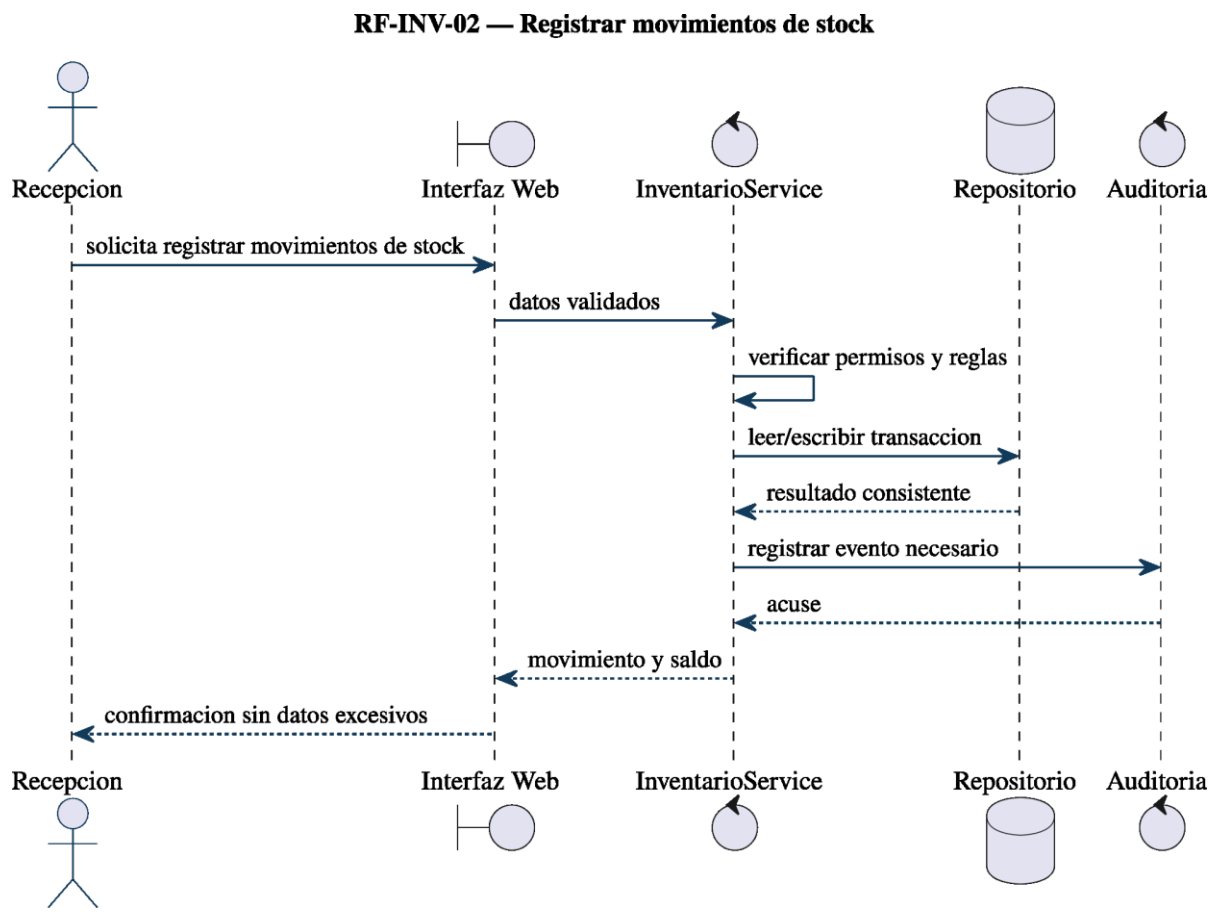
Figura 54: Diagrama de secuencia de RF-INV-02: registrar movimientos de stock.
