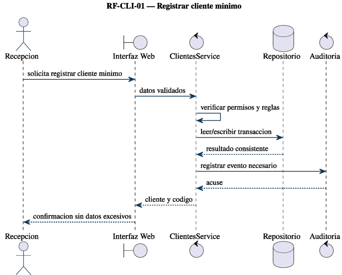
Figura 43: Diagrama de secuencia de RF-CLI-01: registrar cliente minimo.
