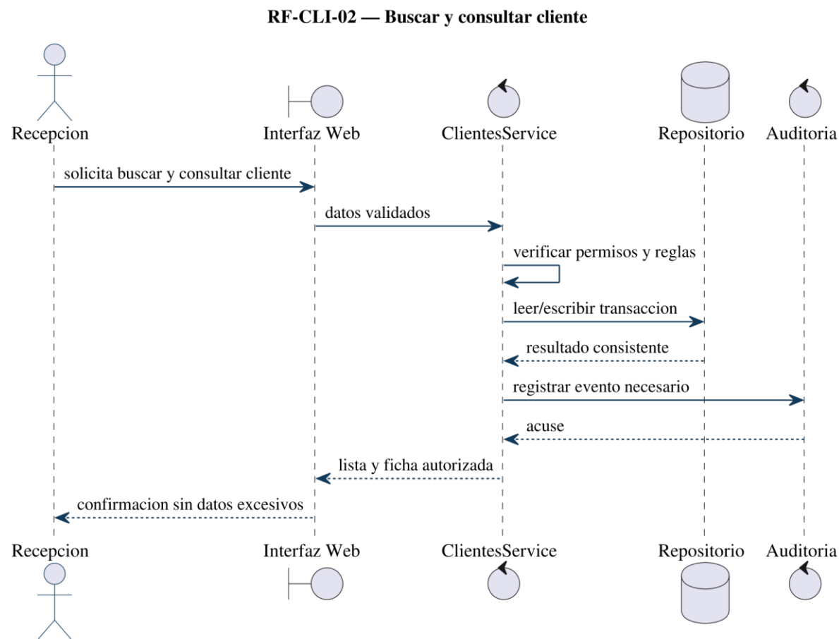
Figura 44: Diagrama de secuencia de RF-CLI-02: buscar y consultar cliente.
