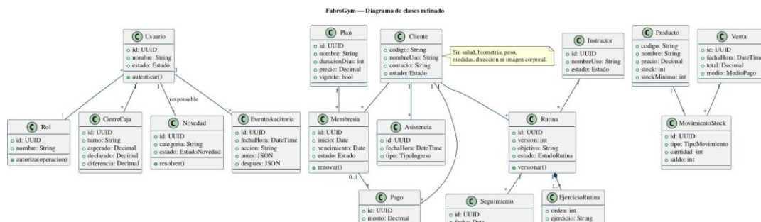
Figura 40: Clases refinadas.
