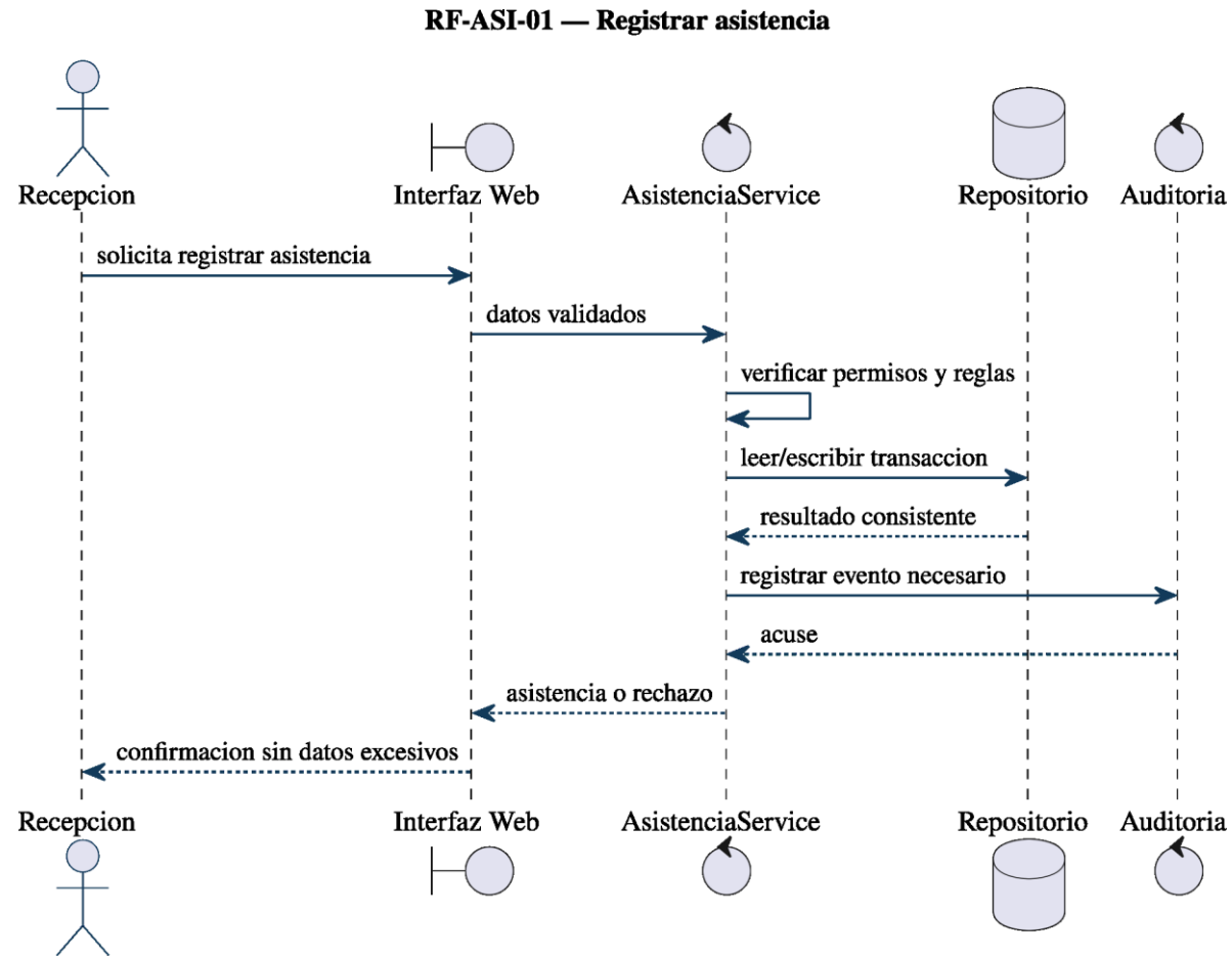
Figura 51: Diagrama de secuencia de RF-ASI-01: registrar asistencia.
