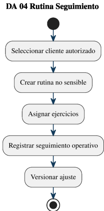
Figura 63: Actividad de rutina y seguimiento.
