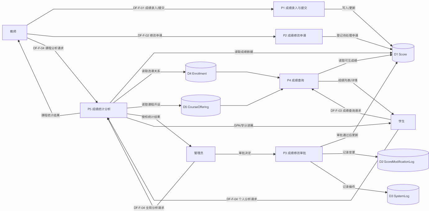
FIG-9-02 F 子系统 0 层 DFD。
