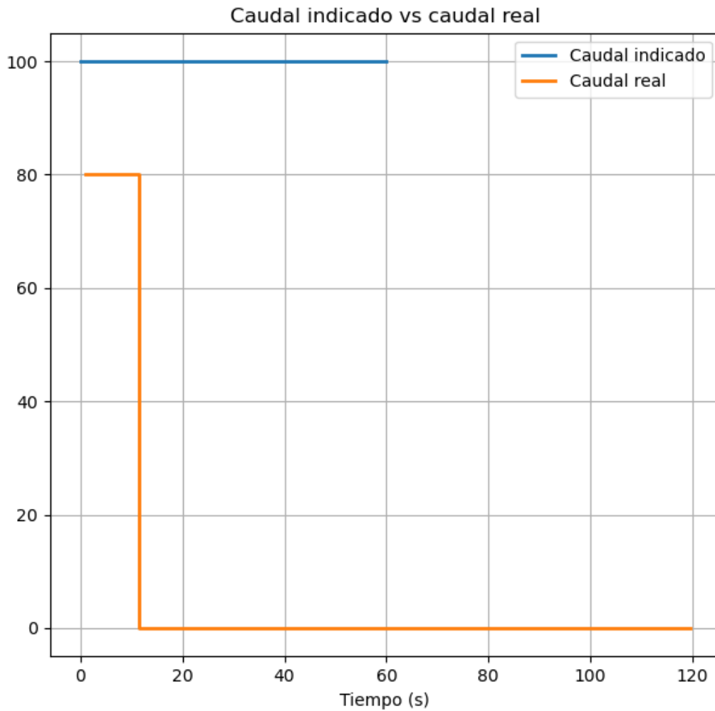
Figura 10: Caudal indicado versus caudal real durante una condición de alarma crítica no confirmada.
