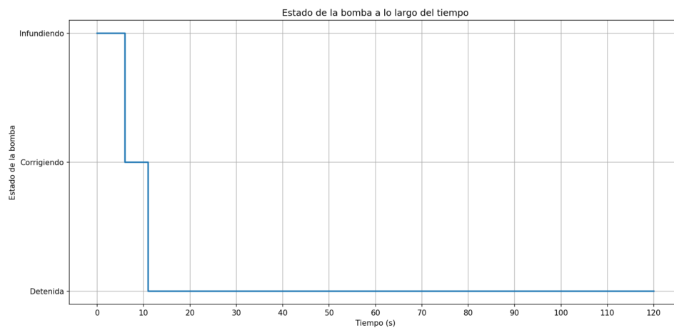
Figura 8: Evolución del estado de la bomba ante un desvío persistente de caudal.
