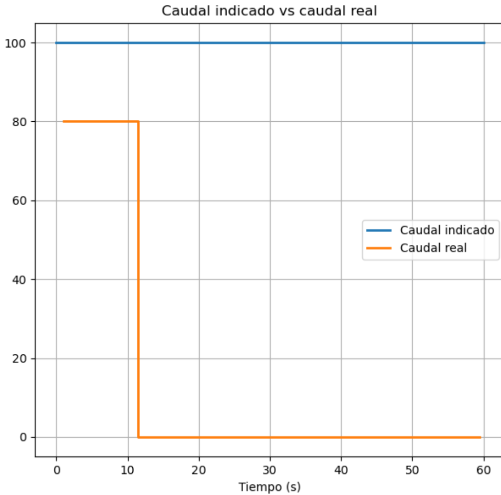
Figura 7: Caudal indicado versus caudal real ante un desvío mayor al 10 %.
