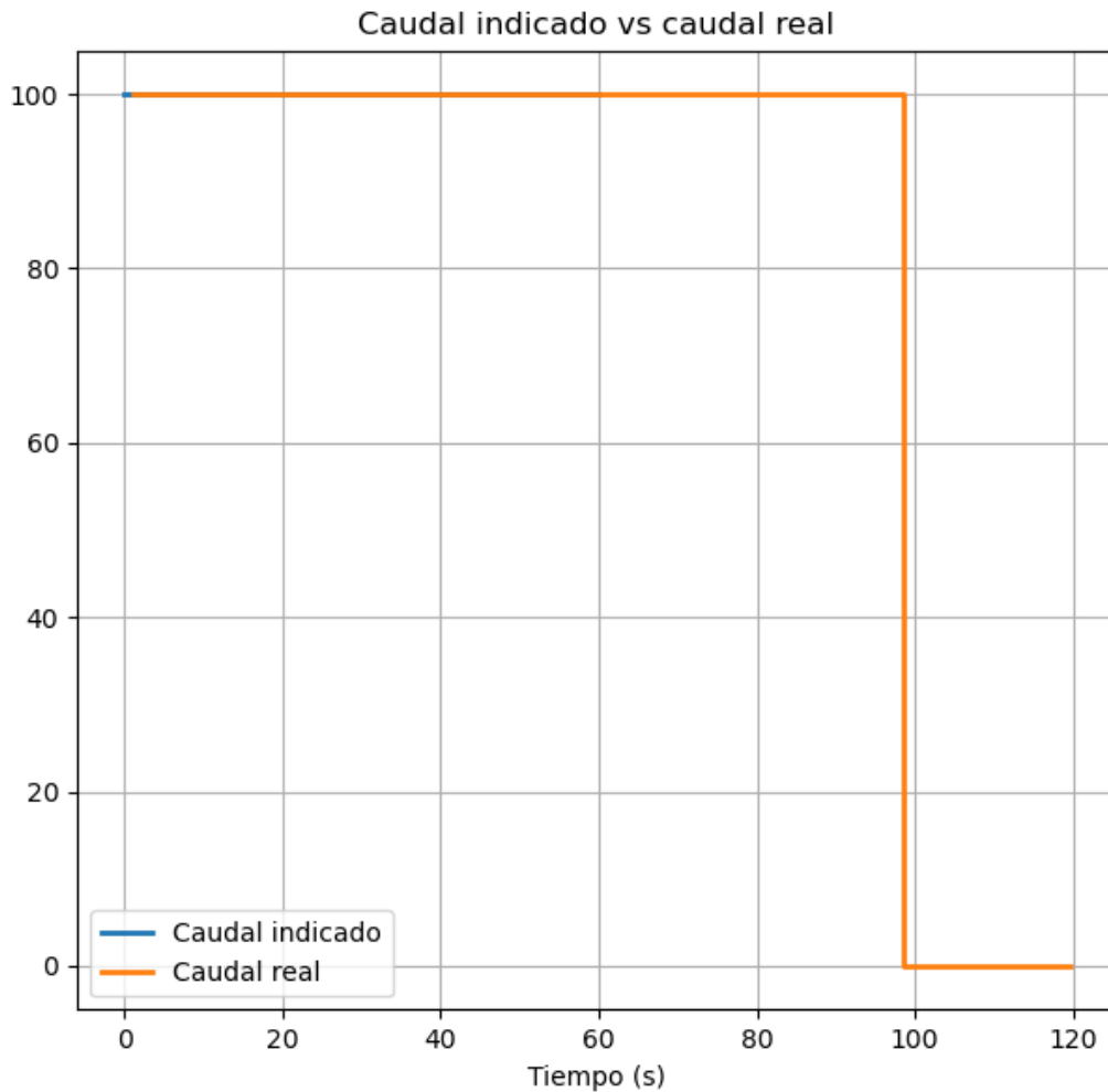
Figura 9: Caudal indicado versus caudal real ante la detección de fin de bolsa.
