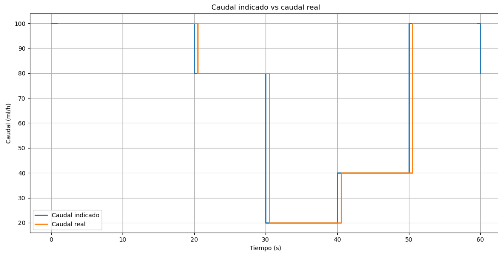
Figura 4: Caudal indicado versus caudal real durante cambios sucesivos de órdenes médicas.
