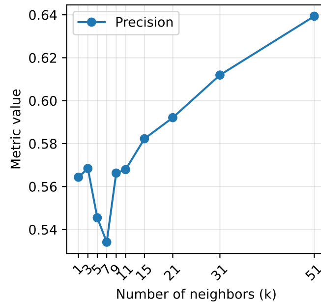
Precision
