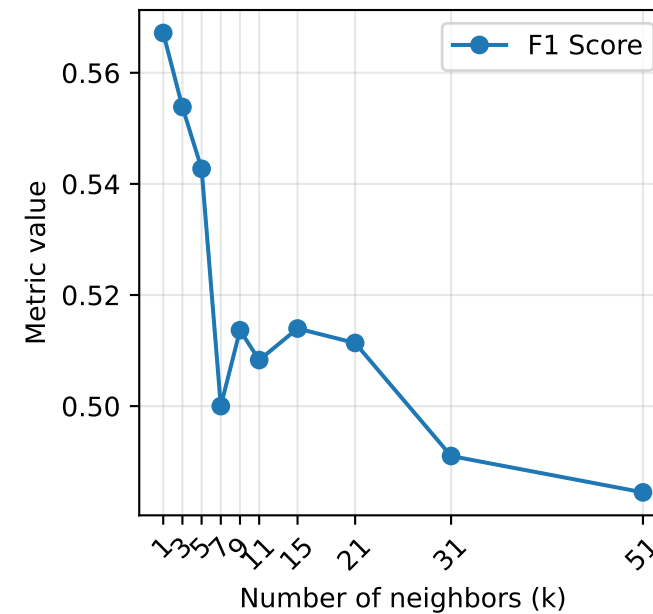
F1 Score
