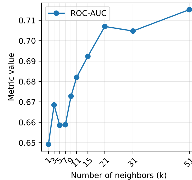
ROC-AUC
