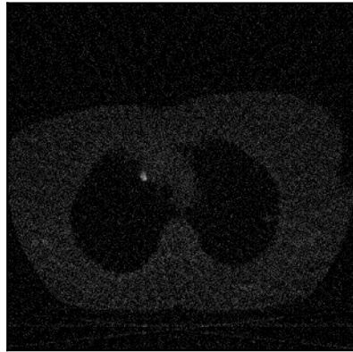
FBP
