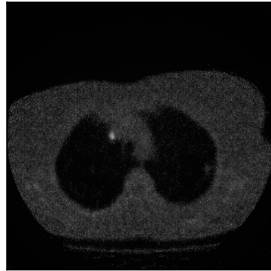
TV
