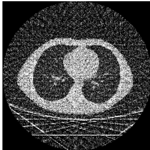
FBP initialisation PSNR = 11.6 dB
