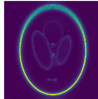
TV-min (30 views)
