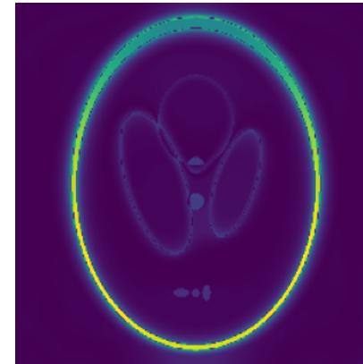
TV-min (720 views)
