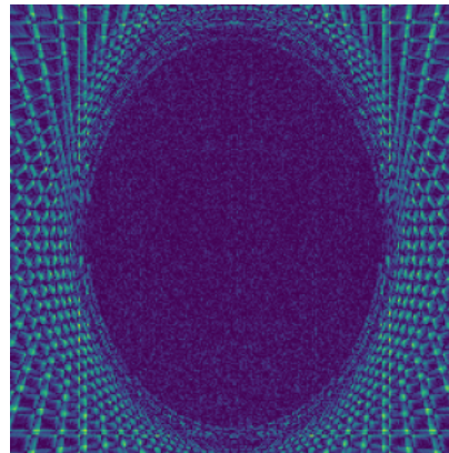
FBP (30 views)
