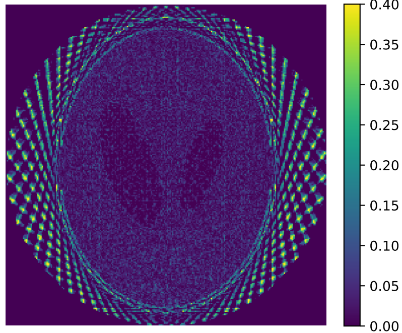
Absolute error
