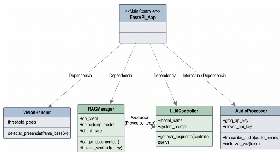
Figura 5: Diagrama de Clases del Backend.
