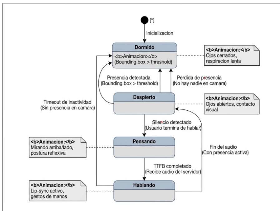
Figura 6: Diagrama de Estados del Avatar.
