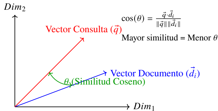
Figura 3: Ilustración geométrica de la Similitud del Coseno en el espacio vectorial RAG.
