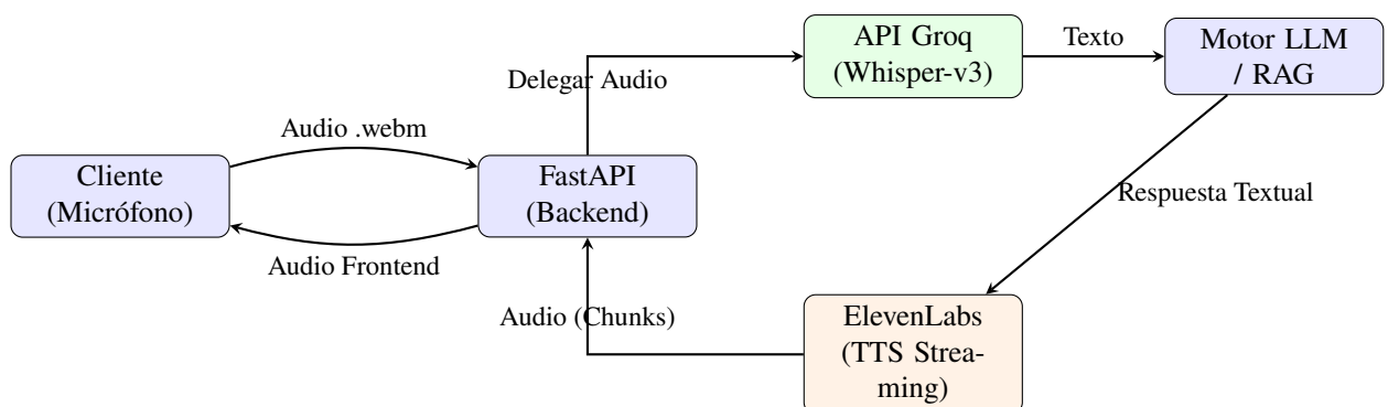
Figura 4: Diagrama de delegación y procesamiento de voz asíncrono en el backend.
