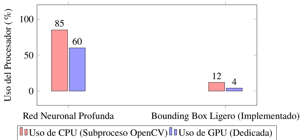
Figura 2: Comparativa del uso de CPU y GPU entre métodos de visión artificial.
