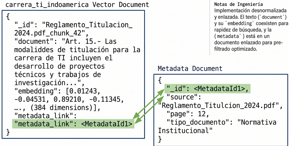
Figura 9: Estructura lógica y proceso de vectorización en la base de datos ChromaDB.
