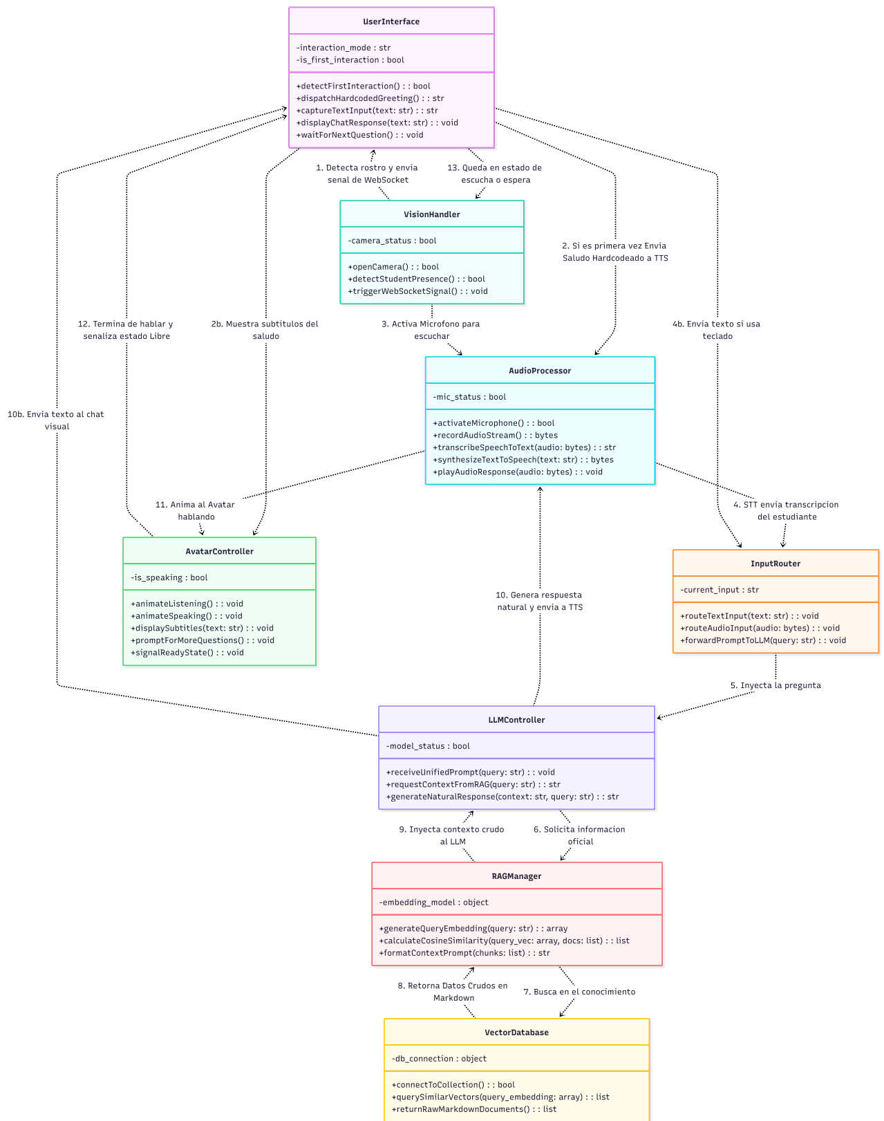
Figura 5: Diagrama de Clases del Sistema (Arquitectura Completa y Flujo Circular).
