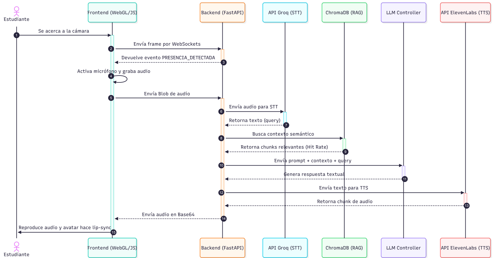
Figura 7: Diagrama de Secuencia de Interacción.
