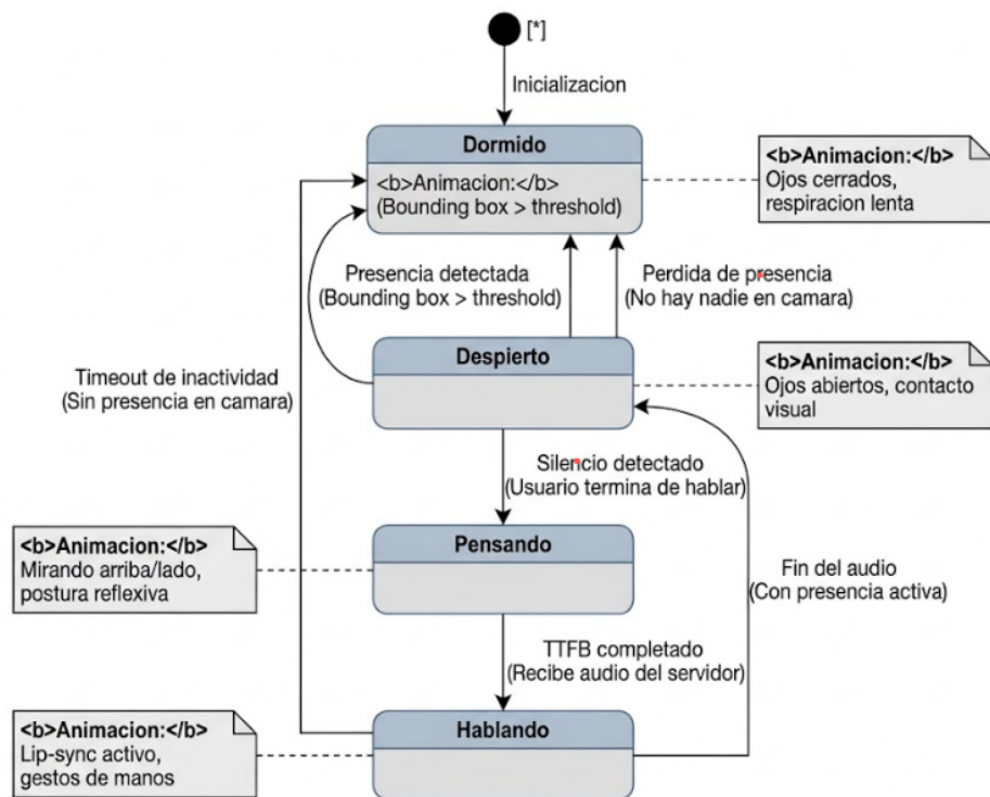
Figura 6: Diagrama de Estados del Avatar.
