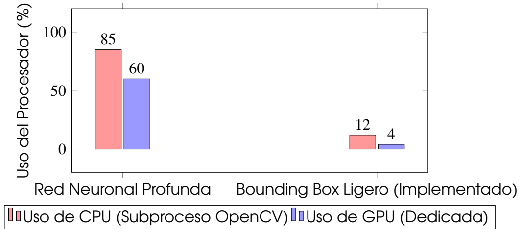
Figura 15: Comparativa del uso de CPU y GPU entre métodos de visión artificial.
