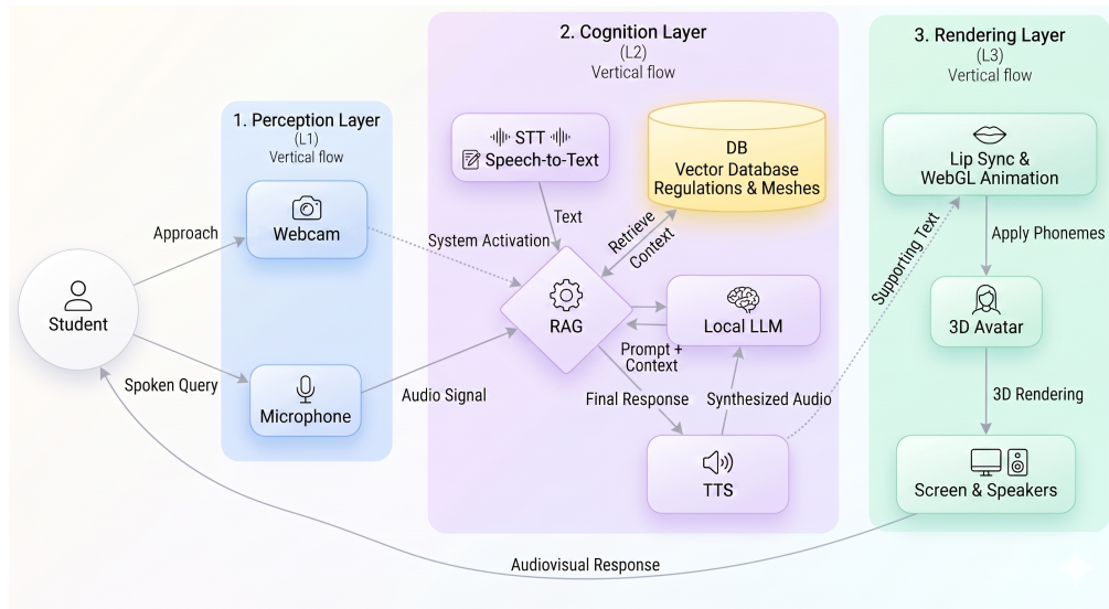
Figura 8: Arquitectura Lógica y flujo de datos del Asistente Virtual (Actualizado).
