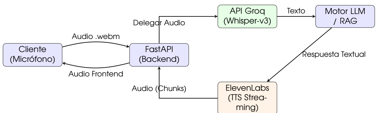
Figura 11: Diagrama de delegación y procesamiento de voz asíncrono en el backend.
