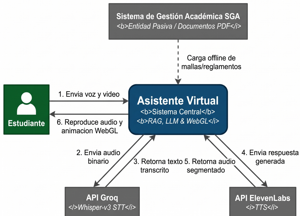
Figura 4: Diagrama de Contexto (Nivel 0).
