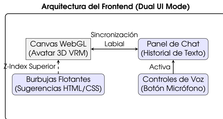
Figura 12: Diagrama de bloques de la Interfaz Dual y composición de elementos web.
