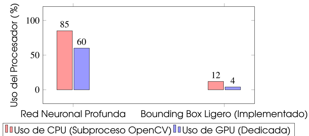
Figura 13: Comparativa del uso de CPU y GPU entre métodos de visión artificial.
