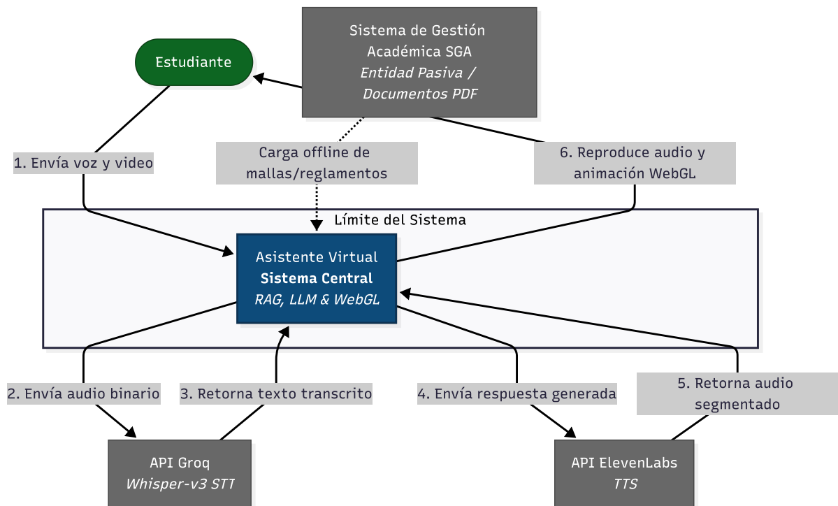
Figura 3: Diagrama de Contexto (Nivel 0).
