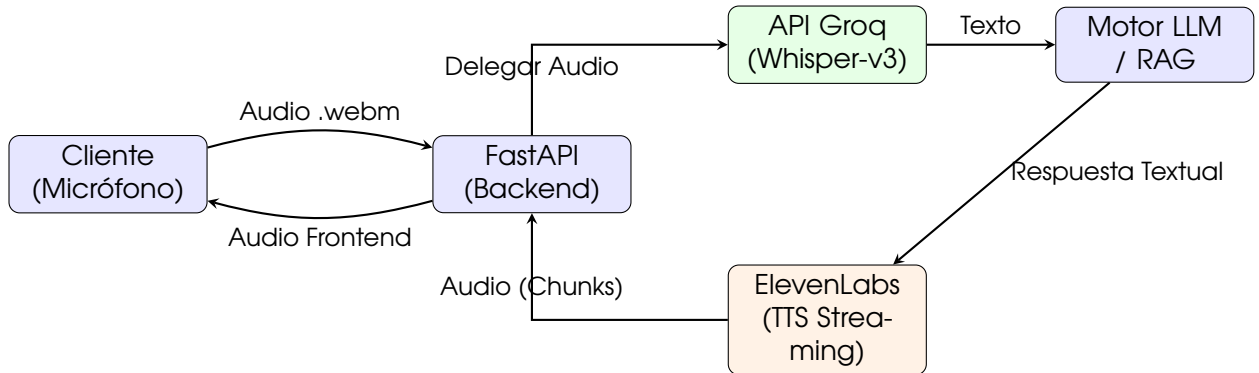
Figura 9: Diagrama de delegación y procesamiento de voz asíncrono en el backend.
