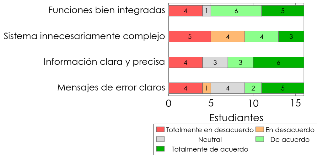
Figura 20: Usabilidad de la interfaz: integración, complejidad (ítem inverso), claridad y mensajes de error.
