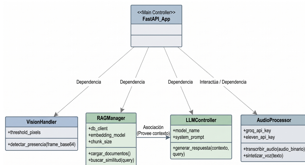
Figura 5: Diagrama de Clases del Backend.
