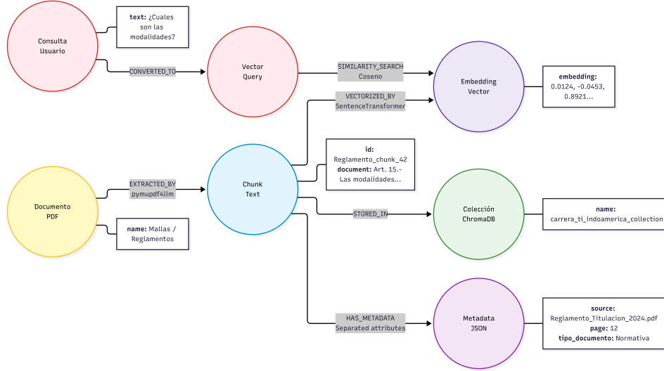
Figura 9: Estructura lógica y proceso de vectorización en la base de datos ChromaDB.
