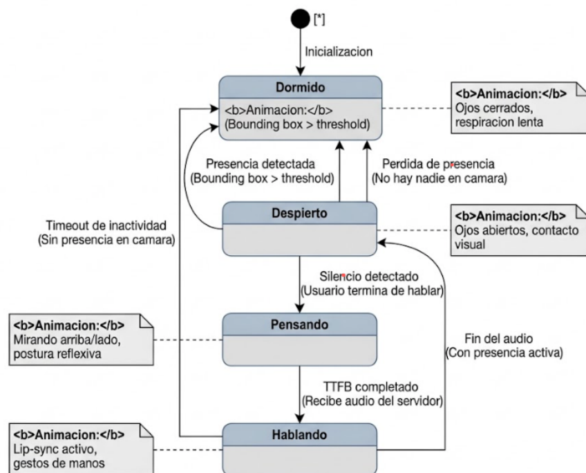
Figura 6: Diagrama de Estados del Avatar.
