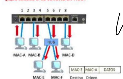
¿Qué sucede si se conecta un HUB?
