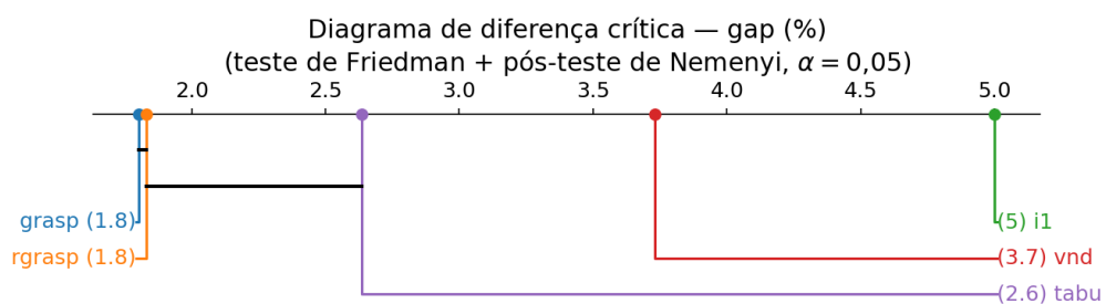
Figure 5 – Diagrama de diferença crítica (Friedman/Nemenyi, 56 instâncias). Cada método aparece na posição do seu rank médio (esquerda = melhor); uma barra horizontal une métodos cuja diferença de ranks é menor que a diferença crítica CD — estatisticamente indistinguíveis a 5%. A leitura correta é dupla: a barra diz quem não se separa; a ausência de barra entre dois métodos diz que a diferença observada dificilmente é acaso.
