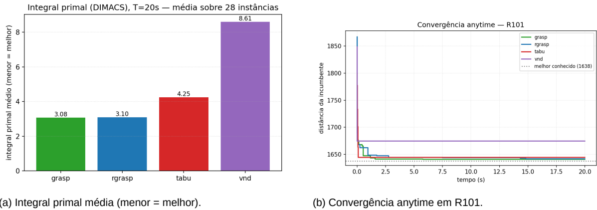
Figura 8 – Análise complementar anytime (integral primal do DIMACS, T = 20 s): métrica dependente de máquina, reportada apenas como complemento.
