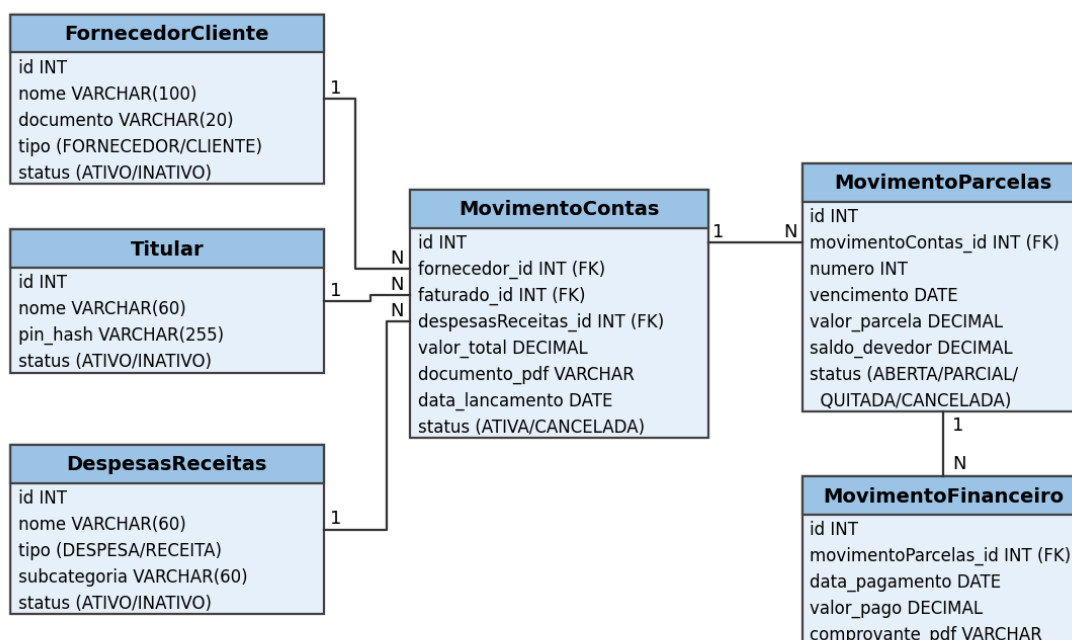
Figura 2 — Diagrama Entidade-Relacional (simplificado).
