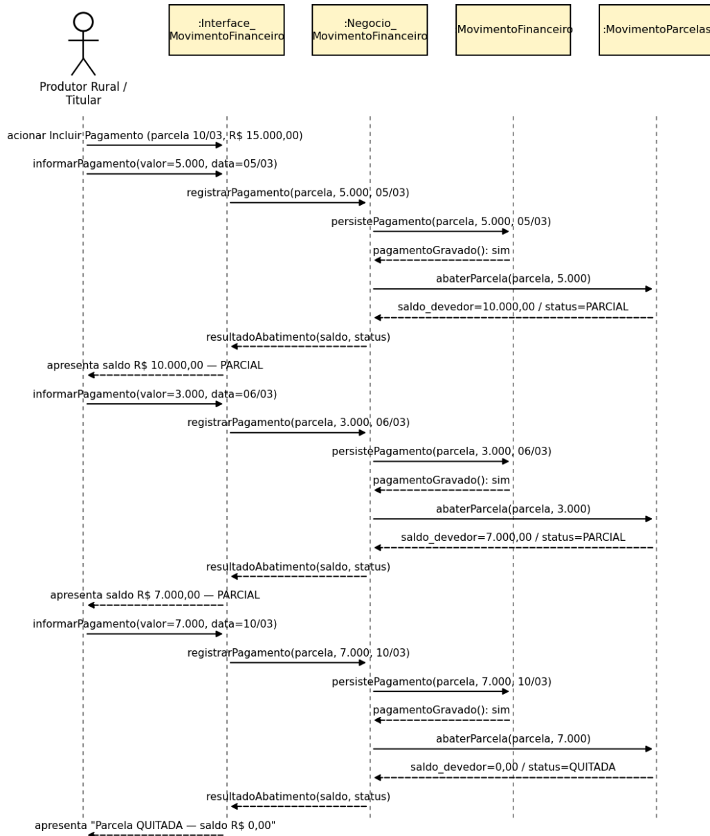
Figura 4 — Sequência do UC05, com os valores reais do exemplo do cliente.
