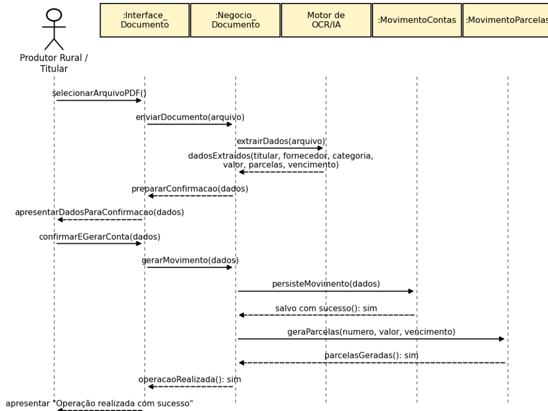
Figura 3 — Sequência dos casos de uso UC06 e UC07.
