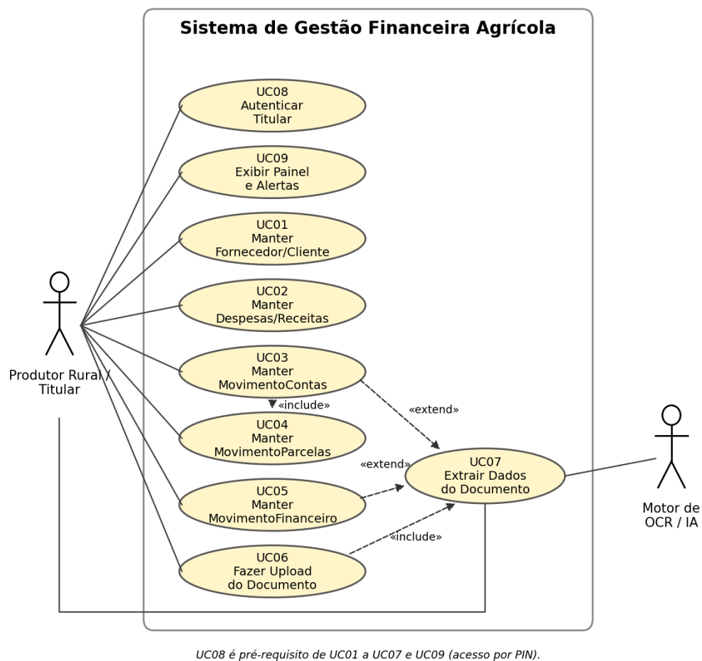
Figura 1 — Diagrama de Casos de Uso do sistema.
