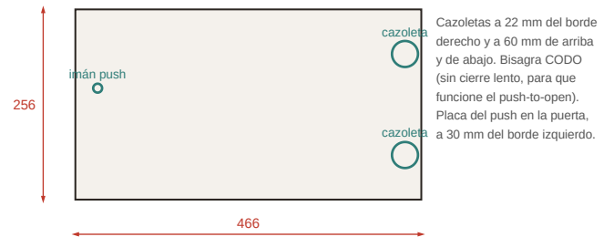
N5 Puerta embutida · nochero
