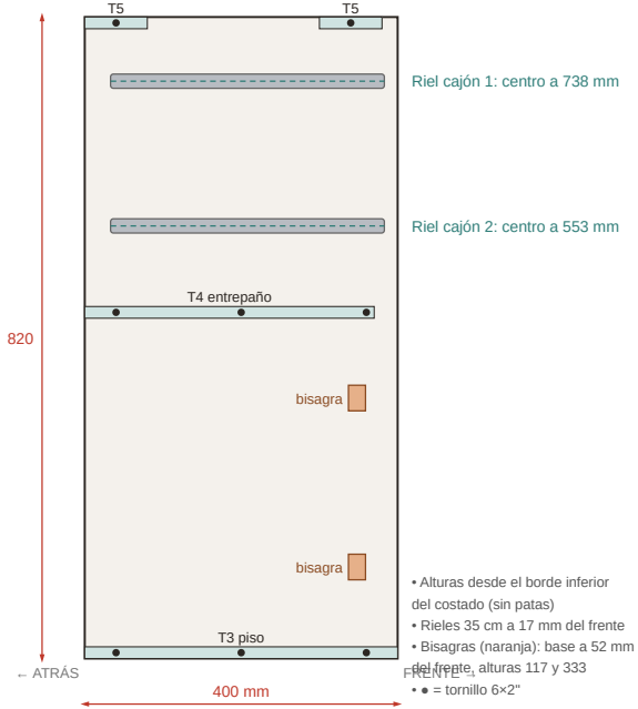
Cómoda Turín · costados (cara interior)
