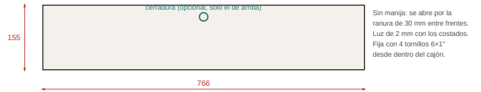
N5 Puerta embutida · nochero
