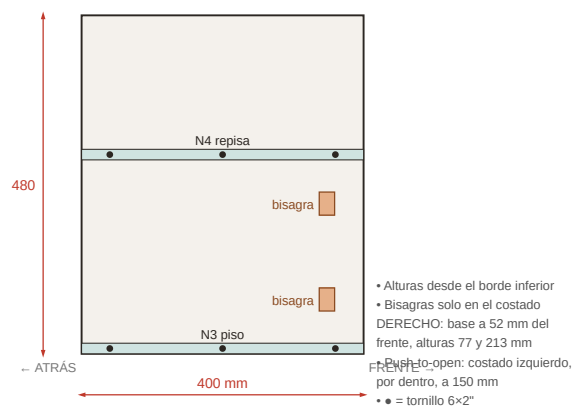
Nochero Sleep · costados (cara interior)
