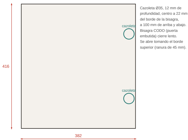
T8 Puerta embutida x2 (derecha; izquierda en espejo)
