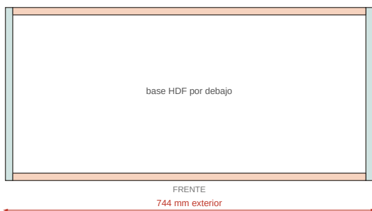
Caja de cajón · Turín (vista superior)
