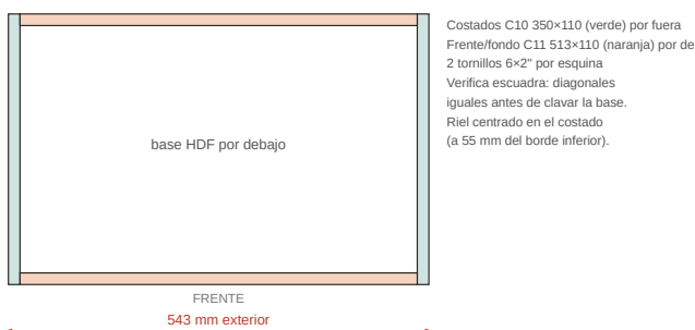
Caja de cajón · cómoda (vista superior)
