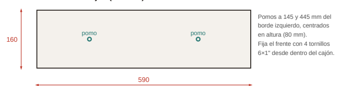
C8 Frente de cajón (cómoda) ×4
