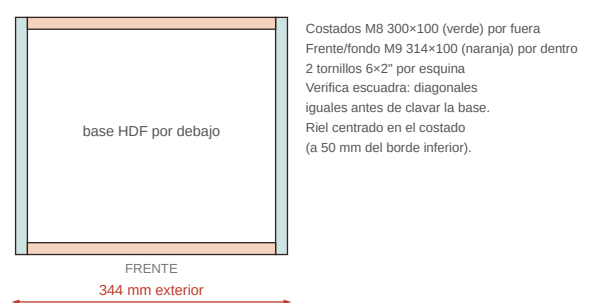
Caja de cajón · mesa (vista superior)
