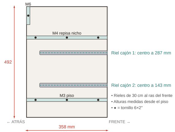
Mesa de noche · costados (cara interior)
