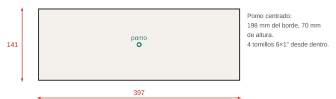
M7 Frente de cajón (mesa) ×2
