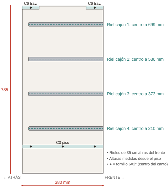
Cómoda · costado izquierdo y división (cara interior)
