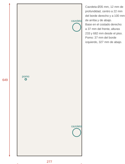
C9 Puerta · cara interior
