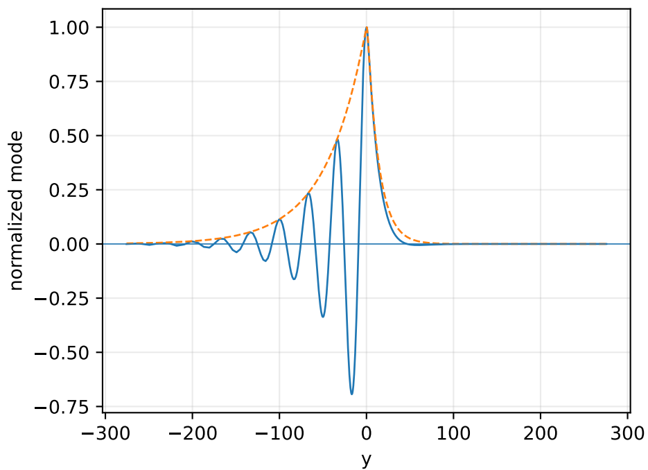
M=1.20, alpha=0.20000 ci=0.063499, N=4593
