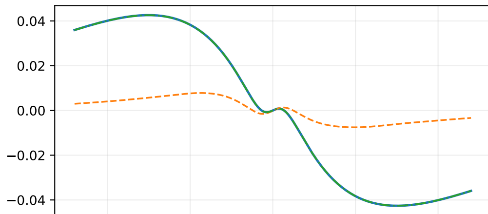
Im ( p )
