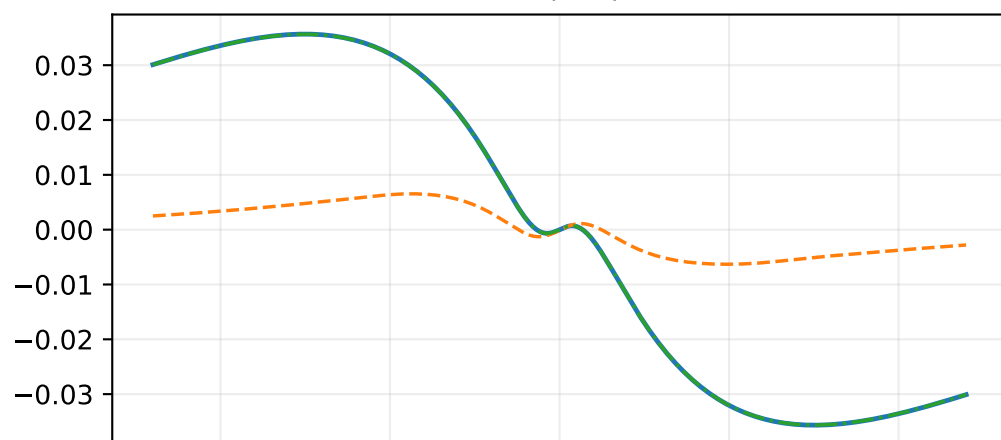
Im ( \rho )
