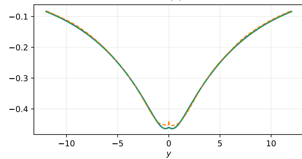
Im ( v )
