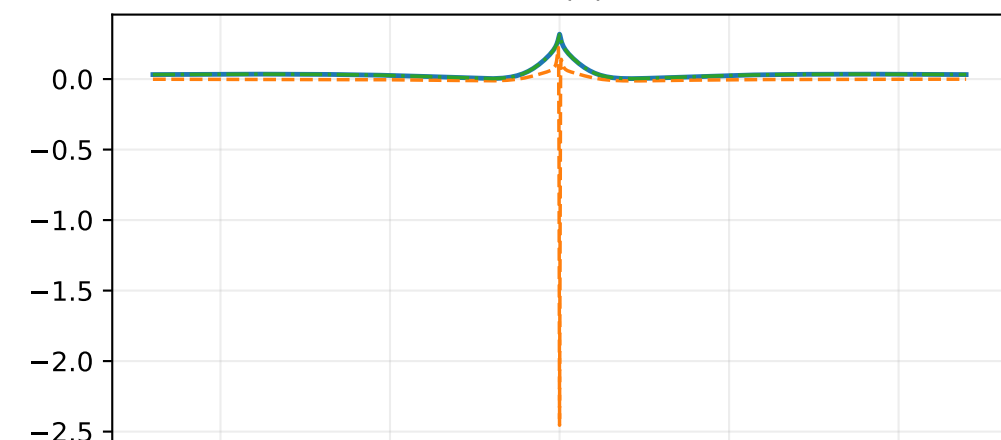
Im ( u )
