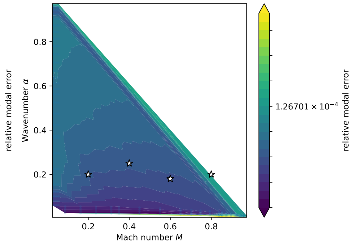
PINN-seeded GEP: v
