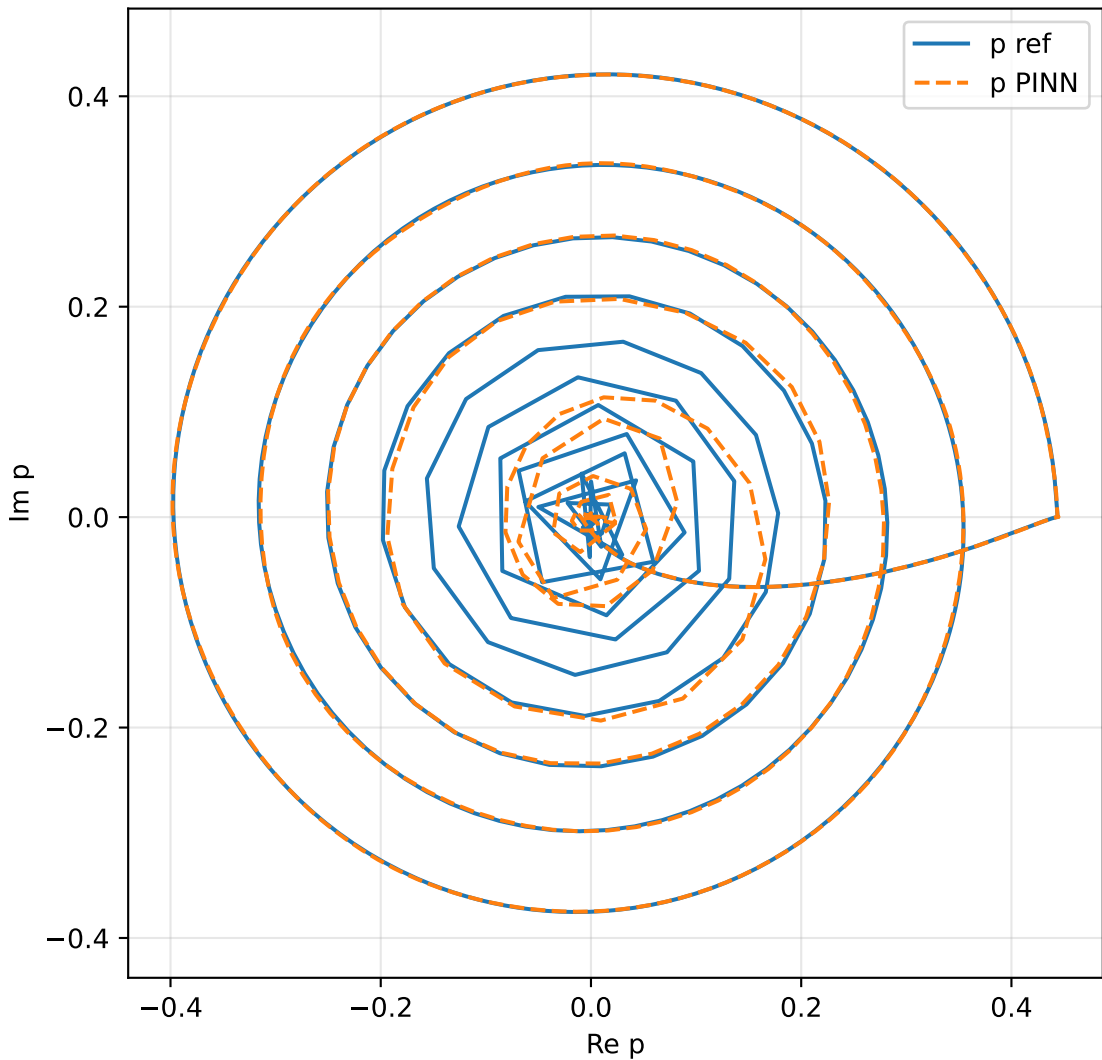
Trajectoire complexe p(y)
