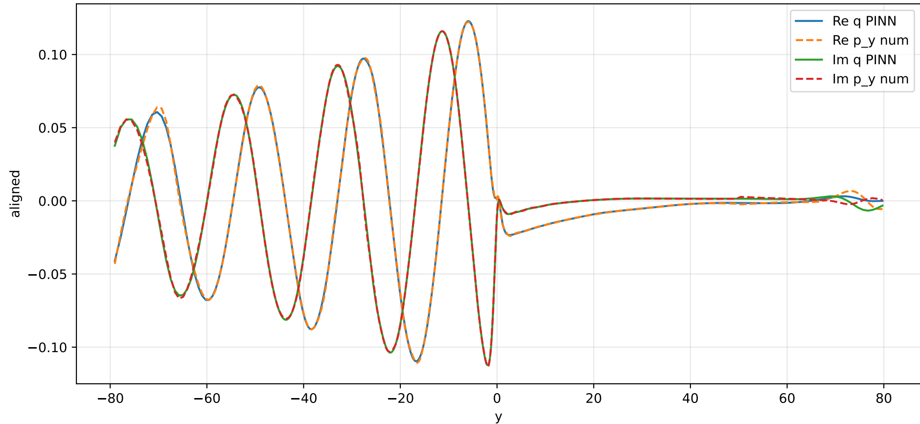
Compatibilité q \approx p_y , centre |y| \leq 80
