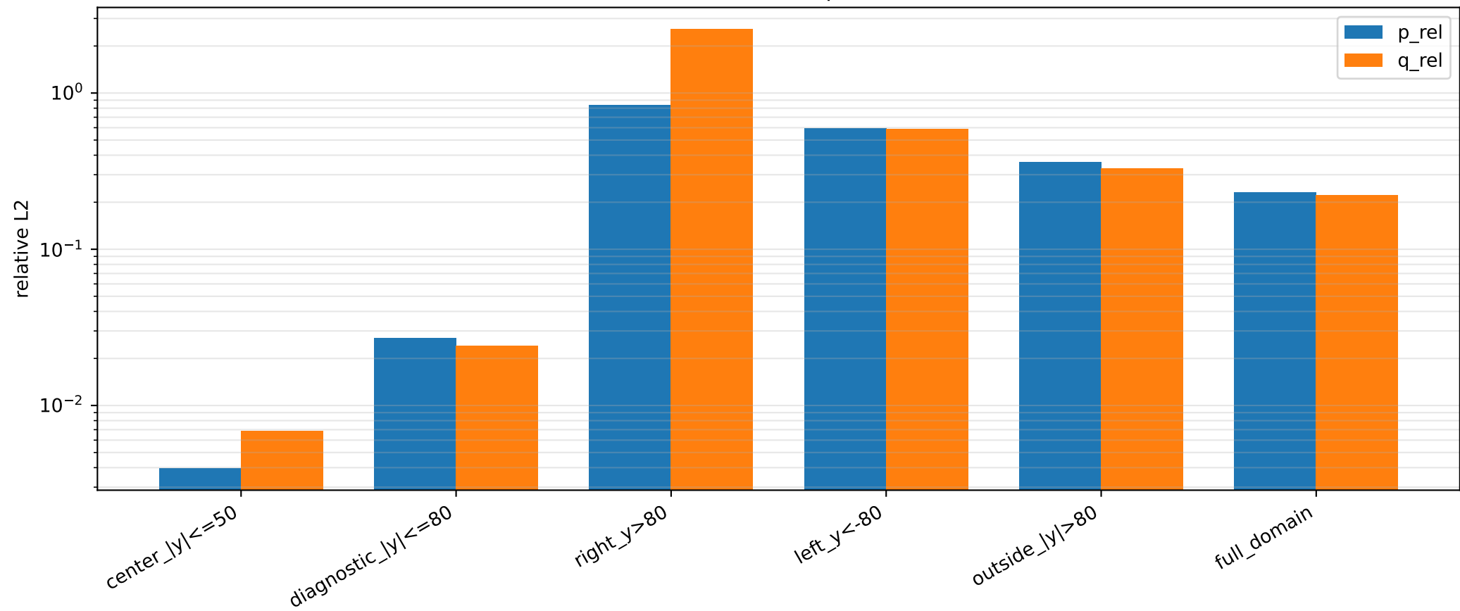
Erreurs relatives par zone
