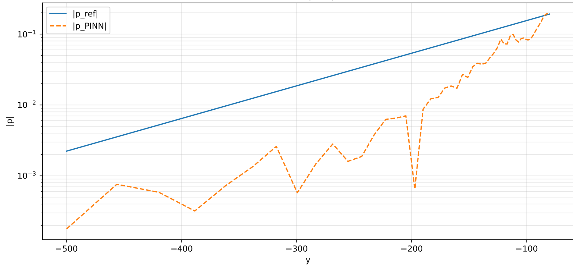
Queue gauche, |p(y)| , y \leq -80
