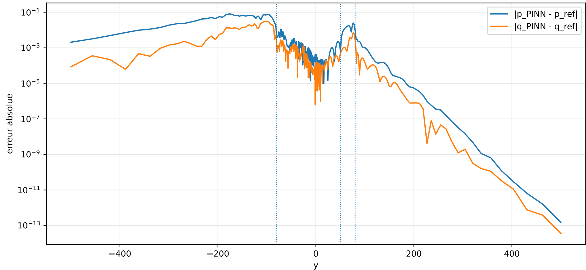
Erreur absolue domaine complet
