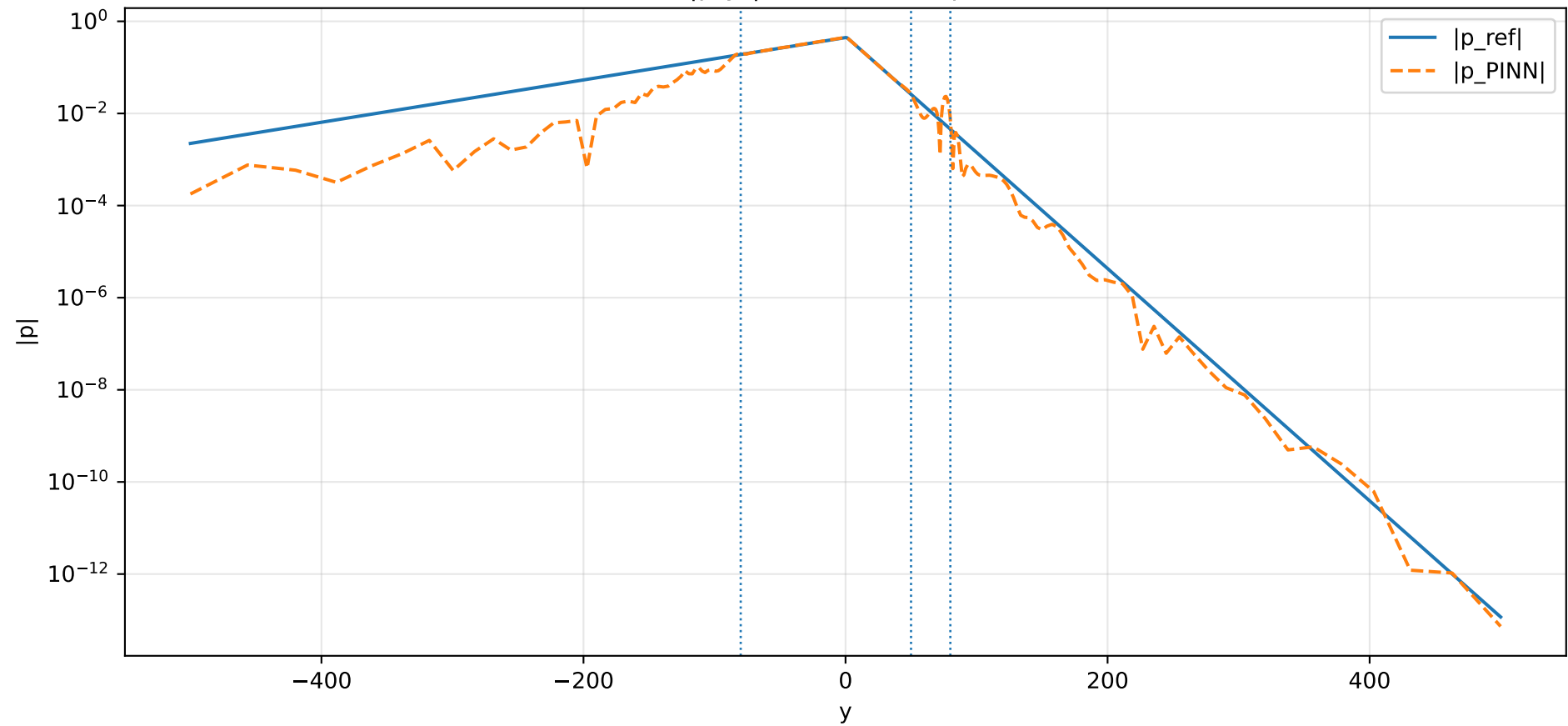
|p(y)| domaine complet
