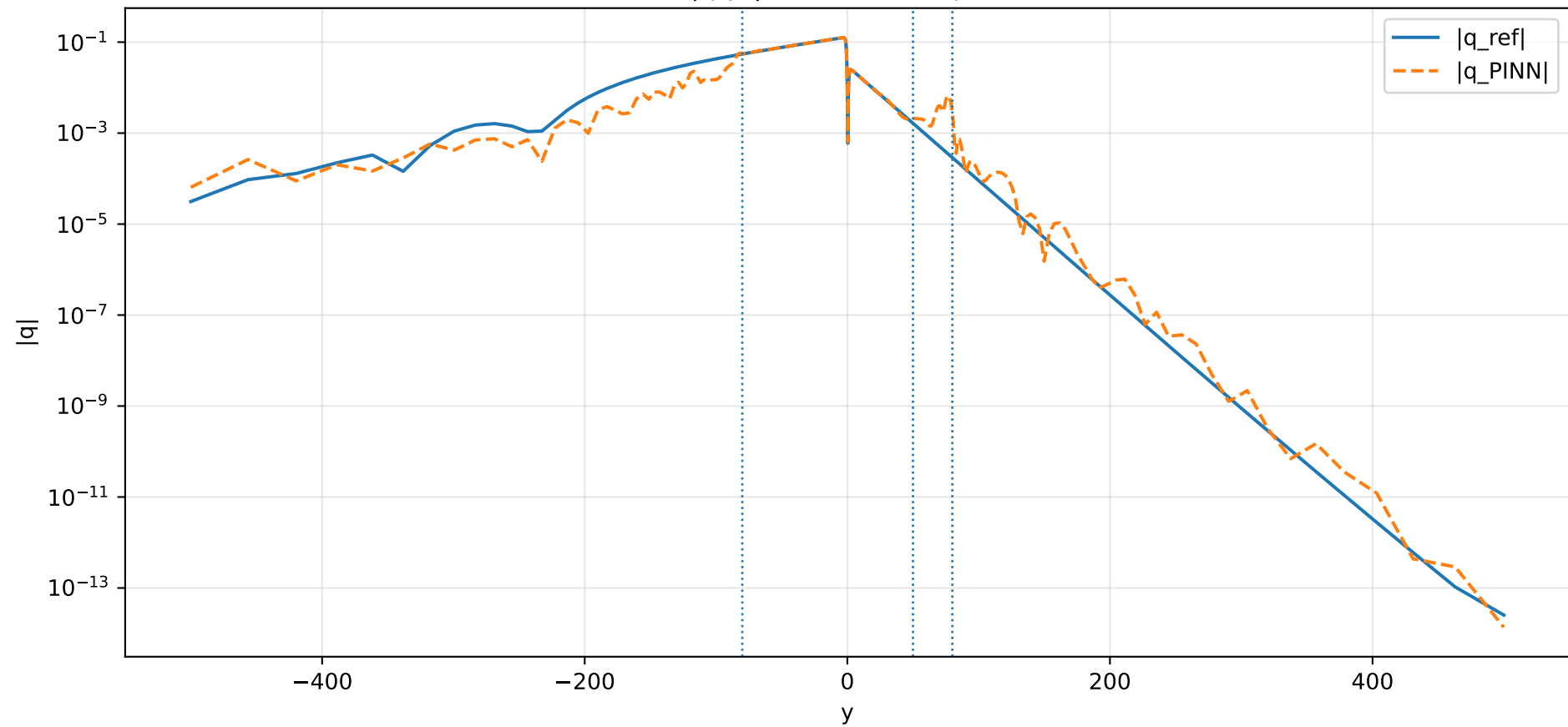
|q(y)| domaine complet
