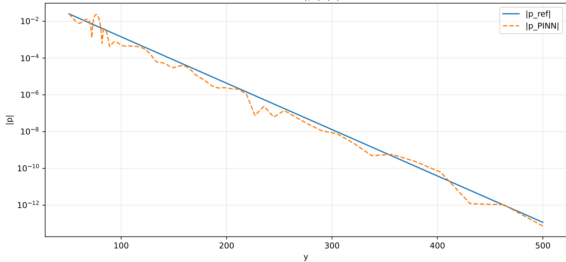
Queue droite, |p(y)| , y \geq 50
